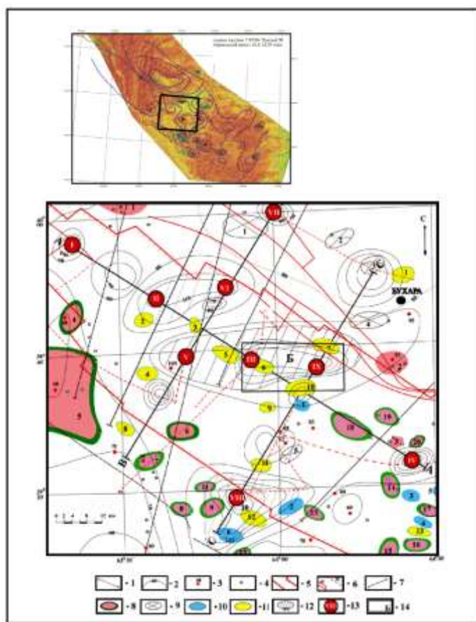
5-расм. Бухоро-Хива палеорифти марказий грабенининг иссиқлик оқими зичлиги харитаси (Тузувчи: У.Н. Рахматов, А.А. Поликарпов, Л.Р. Бикеева маълумотлар асосида, 2021). 1-геотермик съёмка кесма-лари, 2-иссиқлик оқими зичлиги-нинг изолиниялари, 3- ДГС аниқ-ланган учун пунктлар, 4-чуқур кудуқлар, 5-марказий грабен чега-ралари, 6-ёриқлар, 7-сейсмик про-филлар, 8-углеводород конлари, 9-бурғилаш натижалари салбий бўл-ган структуралар, 10-аниқланган структуралар, 11-тайёрланган ту-зилмалар, 12- ДГС аномалиялари, 13-чуқур иссиқлик ва масса узатиш каналлари: I-Тошкудуқ, II-Гўжайли, III-Ғарб. Бештепа, IV-Ғарб. Кўкча, V-Жанубий Гўжайли, VI-Муродкудуқ, VII-Отбоқар, VIII-Тегирмон, IX-Чуқуркўл, 14- дала термобарогеокимёвий съёмка участкаси.
