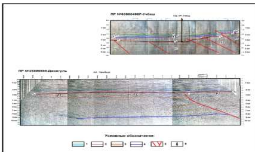
Рис.3. Система поперечных сейсмо-геологических разрезов цент-рального грабена Буха-ро-Хивинско-го палеориф-та по про-филям метод общей глу-бинной точки в двухмерном варианте №63 980496Р-Уч-баш и №2589 0688-Джан-гуль (Соста-вил: Рахматов У.Н. с ис-пользованием материалов Гафурова Т.А., Эгамова В.С., Максудова М.Х., Сафонова Б.К., Криц Б.А., Колес-ниченко Л.Ю., 2020 г.). 1 - опорные отражающие горизонты, 2 – поверхность палеозойского комплекса, 3 – отражающие границы внутри палеозойского комплекса, 4 – поверхность дорифтового палеозойского комплекса, 5 – разрывные нарушения, 6 – глубокие скважины.
