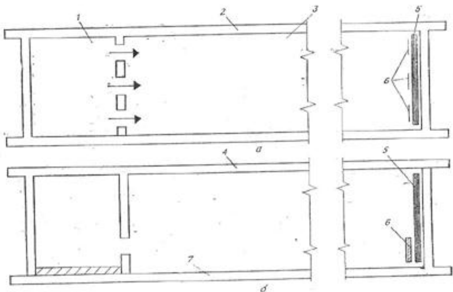
3-расм. Ёпиқ типдаги тир схемаси
