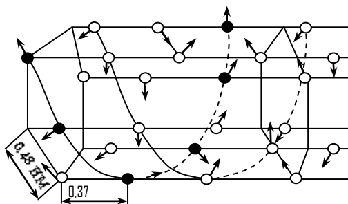
1-расм. Карбамид комплекси кристаллик панжараси схемаси.
