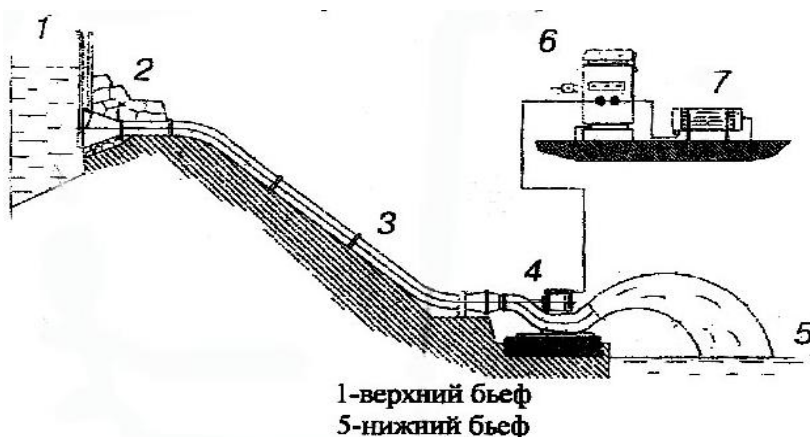
Рис. 2.6. Схема установки микроГЭС.
