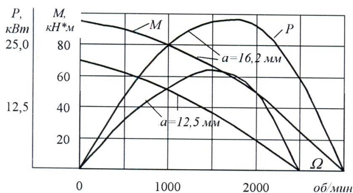
Рис. 2.11 Характеристики гидротурбины типа К-245, D=289 мм, H=9 м
