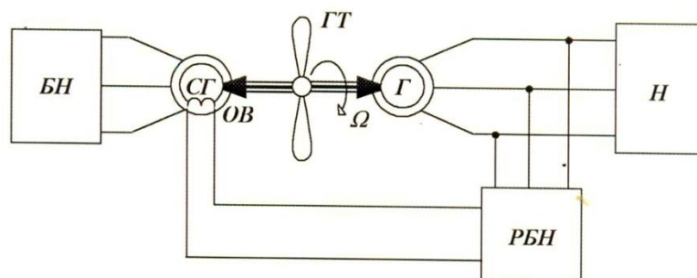
Рис.2.2 Структурная схема микроГЭС автобалластного типа, построенная на базе двух генераторов
