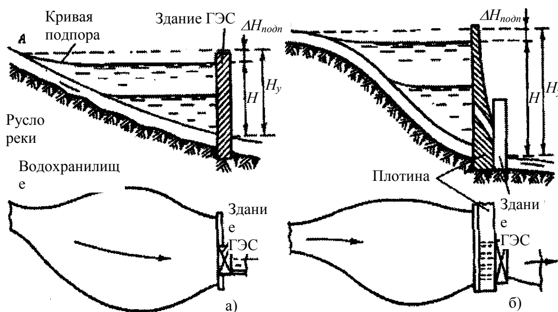
Рис. 2.1 Плотинные схемы концентрации напора
