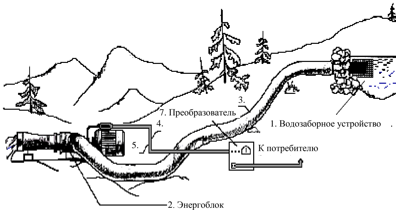
Рис. 4.1. Установка для использования энергии малых водотоков
