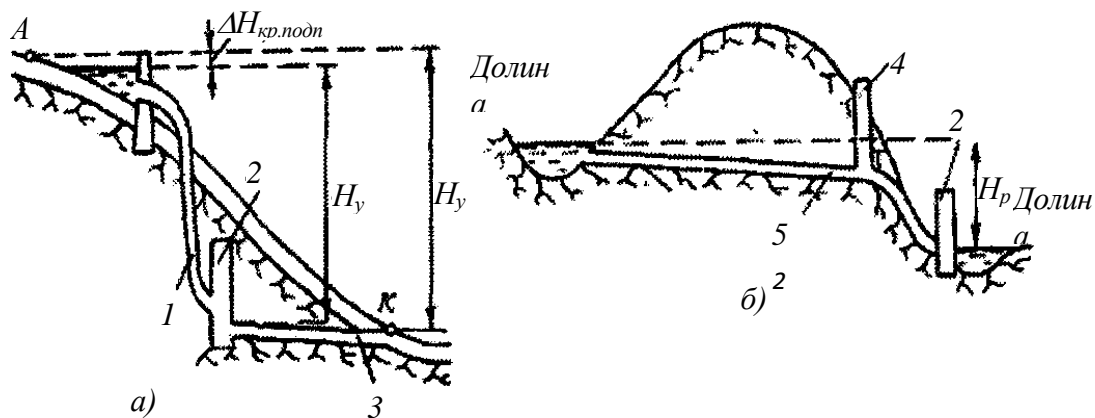
Рис. 2.3 Другие схемы концентраций напора.
