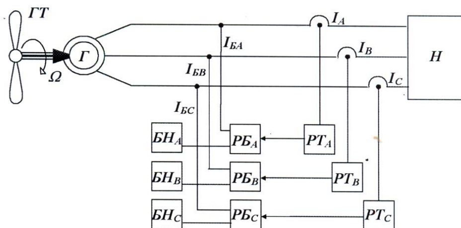
Рис. 3.5 Структурная схема микроГЭС с управлением по току нагрузки
