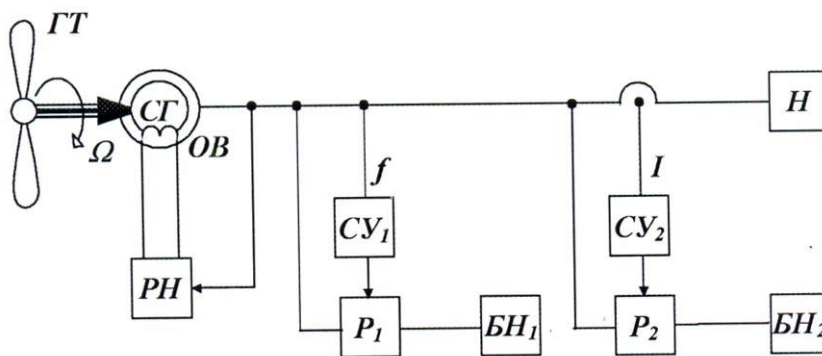
Рис. 3.6 Структурная схема микроГЭС с комбинированной системой управления
