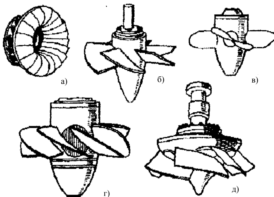
Рис.2.4 Общий вид рабочих колес реактивных турбин.
