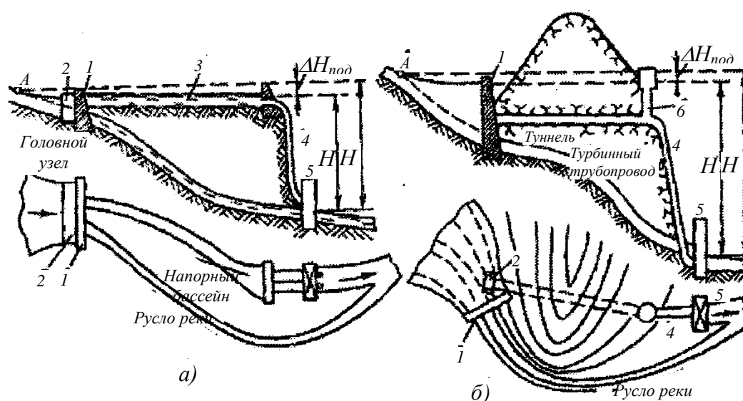
Рис. 2.2 Деривационные концентрации напора а) с безнапорной деривацией; б) с напорной деривацией; 1-плотина; 2-водоприемник;
