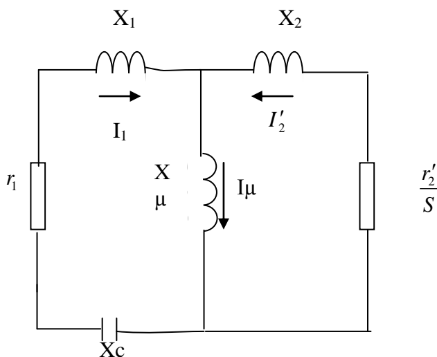
Рис.4.2.Эквивалентная схема асинхронной машины при конденсаторном торможении
