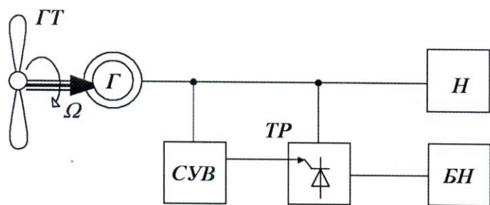
Рис. 3.4 Структурная схема микроГЭС с фазовым управлением
