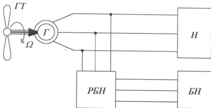
Рис. 3.1 Структурная схема стабилизации параметров микроГЭС автобалластного типа
