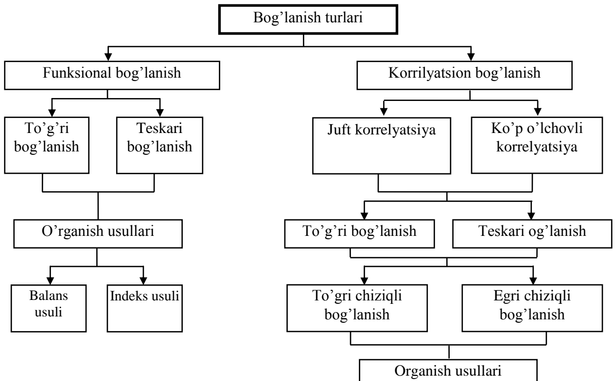
10.1-tarh. Hodisalar orasidagi o'zaro-bog'lanish turlari va o'rganish usullari.
