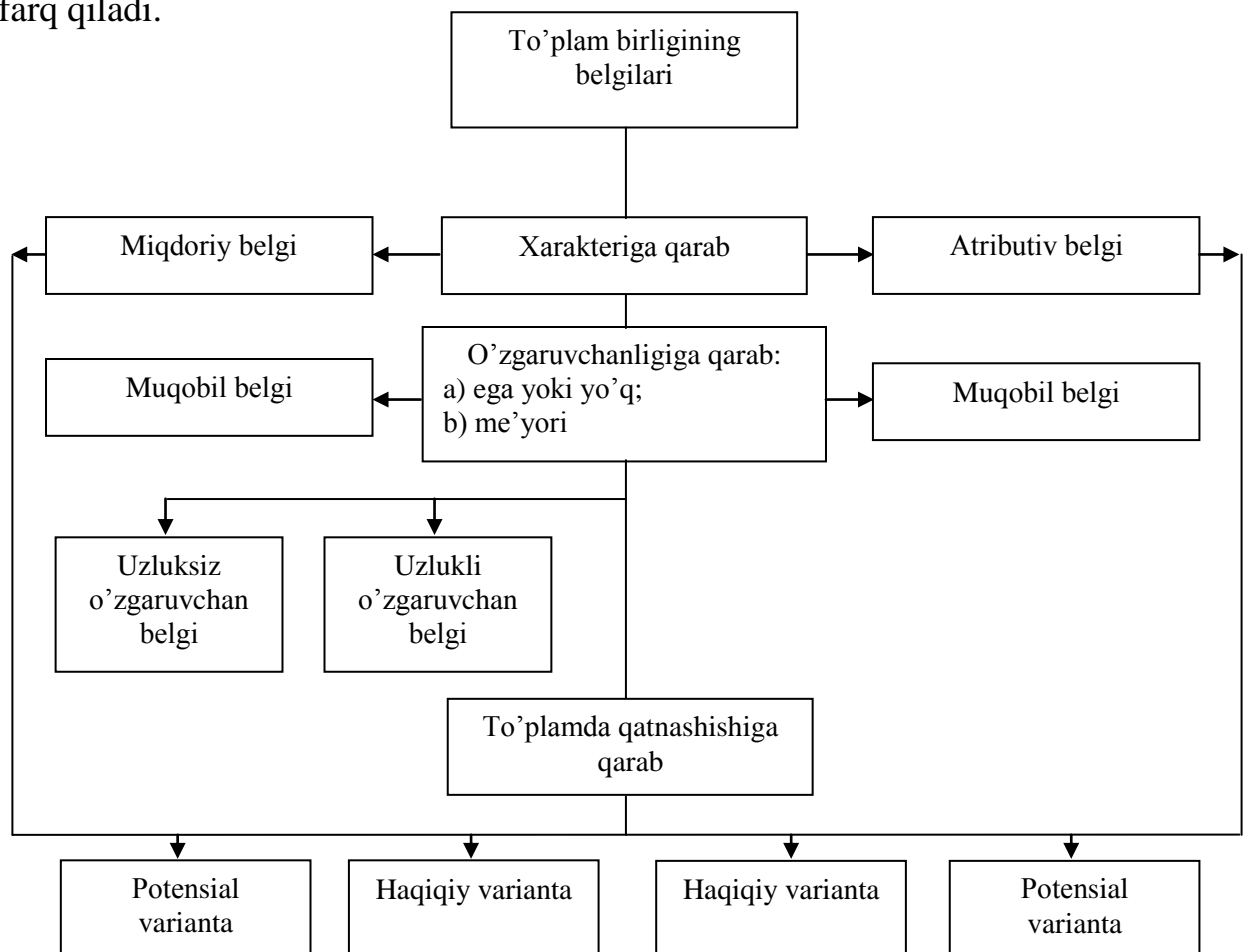
6.1-tarh. To‘plam birligi belgilarining turlari.
