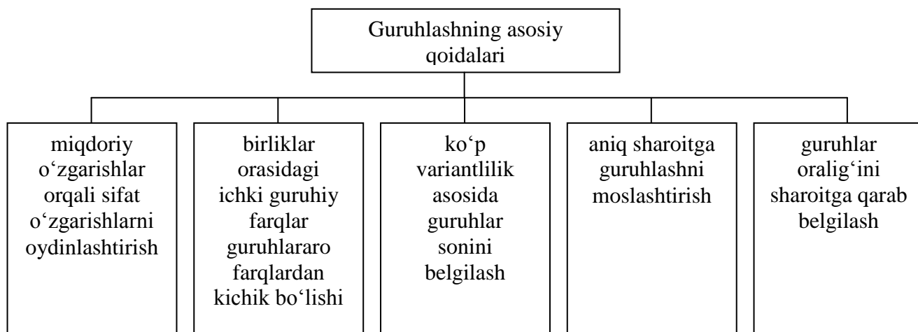
5.1.-tarh. Guruhlashning asosiy qoidalari.
