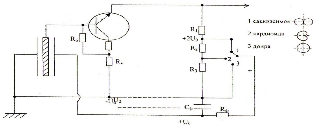
2.3-расм. Комбинацияланган конденсаторли микрофон тузилишининг бир кўриниши.
