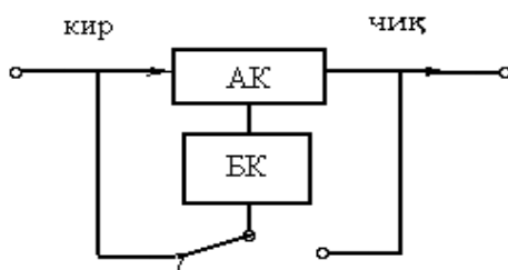
1.6-расм. Автоматик сатх бошқаргичларининг умумлаштирилган схемаси.
