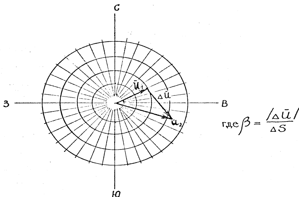
Векторная диаграмма сдвига ветра \bar{u}_1 и \bar{u}_2 — векторы скорости ветра, измеренные в двух точках пространства; \Delta \bar{u} — вектор сдвига ветра; \Delta S — расстояние между двумя точками в пространстве.
