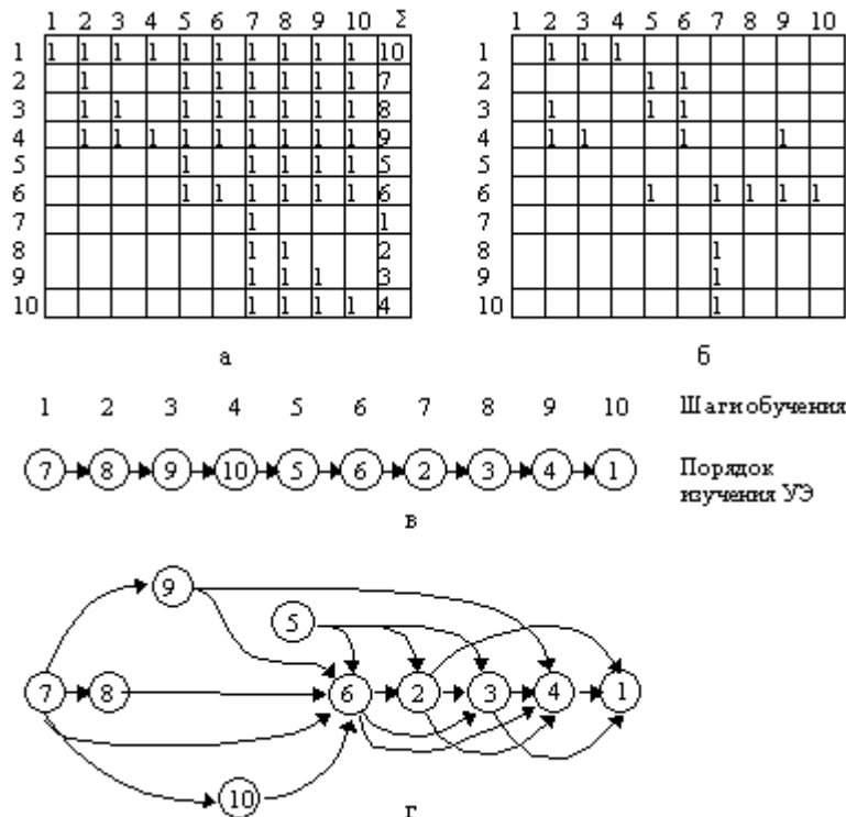
Рис. 2.4.1. Пример модели освоения учебного материала:
