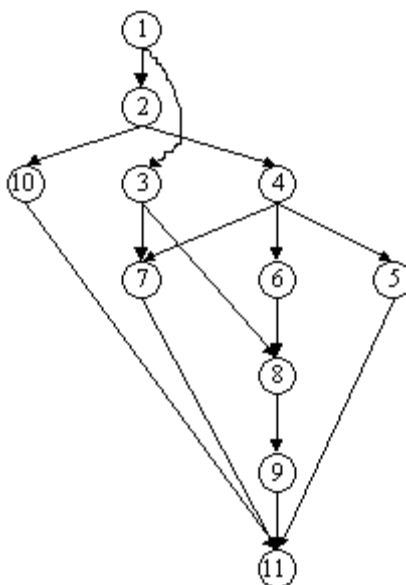
Рис. 2.4.5. Сокращенный граф логических связей.
