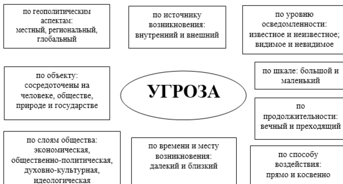
Рисунок 1. Классификация угроз
