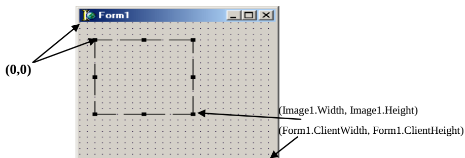
1-расм. Чизиш юзаси нуқта координаталари.
