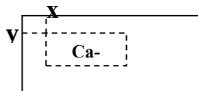
3-расм. Матн ҳосил бўлувчи соҳа координатаси
