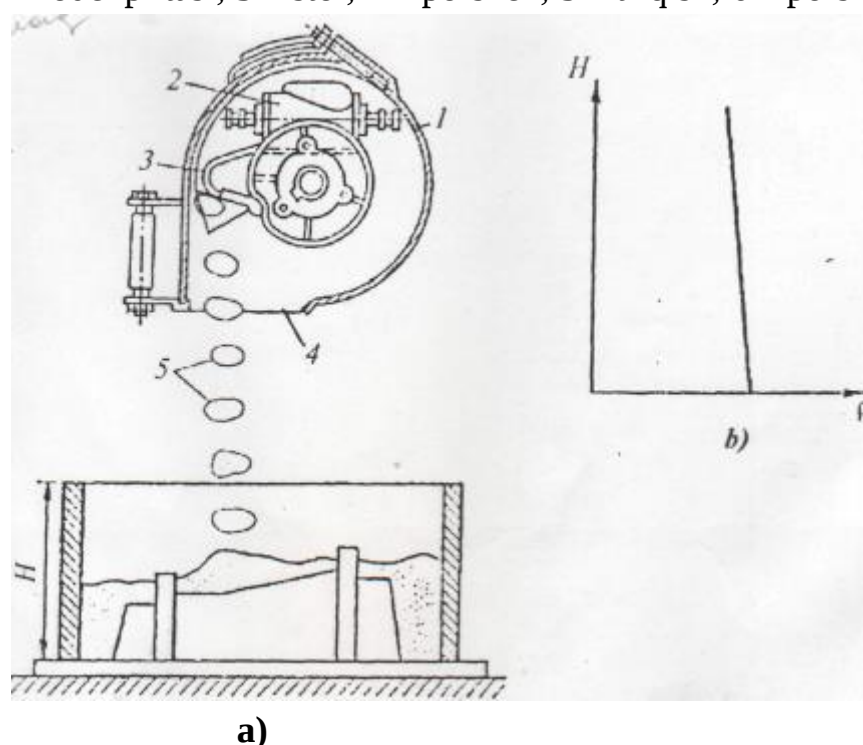
25rasm. Qumotar kallagi yordamida qolipni zichlash va opokaning balandligiga qarab zichligining o'zgarishi:
