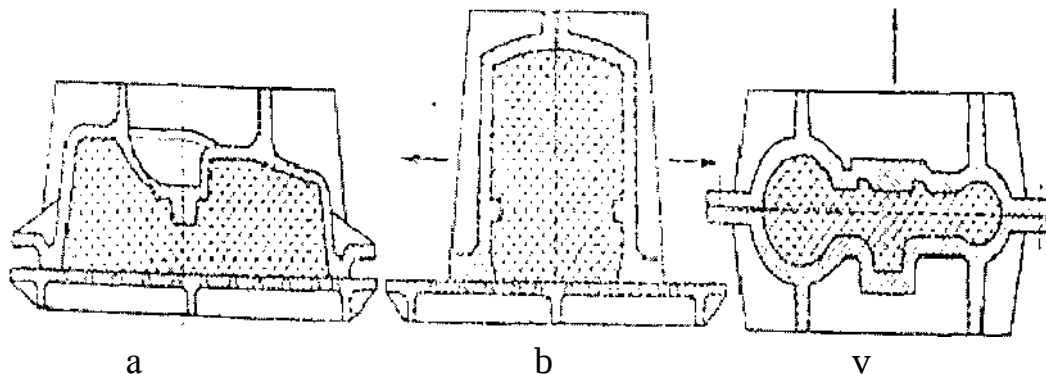
5- rasm. Metalldan ishlab chiqilgan qutilar: a – qoqib chiqaradigan; b – vertikal ajralish chiziqli; v – gorizontal ajralish chiziqli
