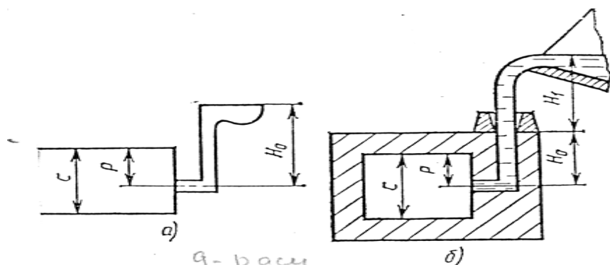
14-rasm. a, b rasmlarga ko'ra quyuv sistemalari uchun
