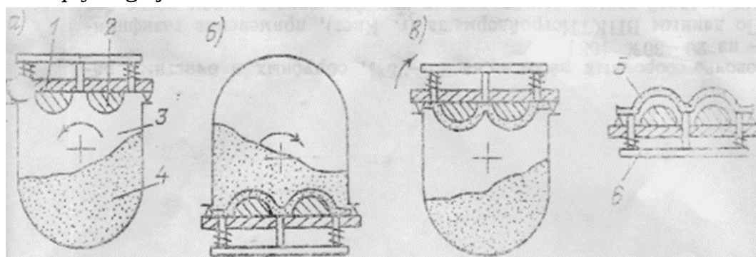
36-rasm. Qobiq qolipda quymani tayyorlab olish sxemasi:
