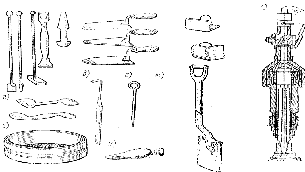
20-rasm. Qolipni tayyorlab olishda ishlatiladigan asbob – uskunalar:
