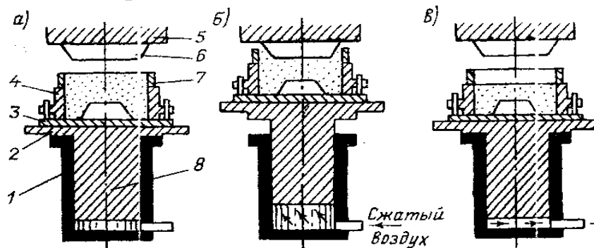
23.2-rasm. Yuqoridan presslash mashinani ishlash sxemasi
