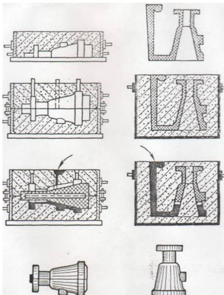
35-rasm. Gazlanib chiqib ketadigan moslama yordamida quymani olish sxemasi: a – oddiy usulda; b – gazlanib chiqib ketadigan moslama yordamida
