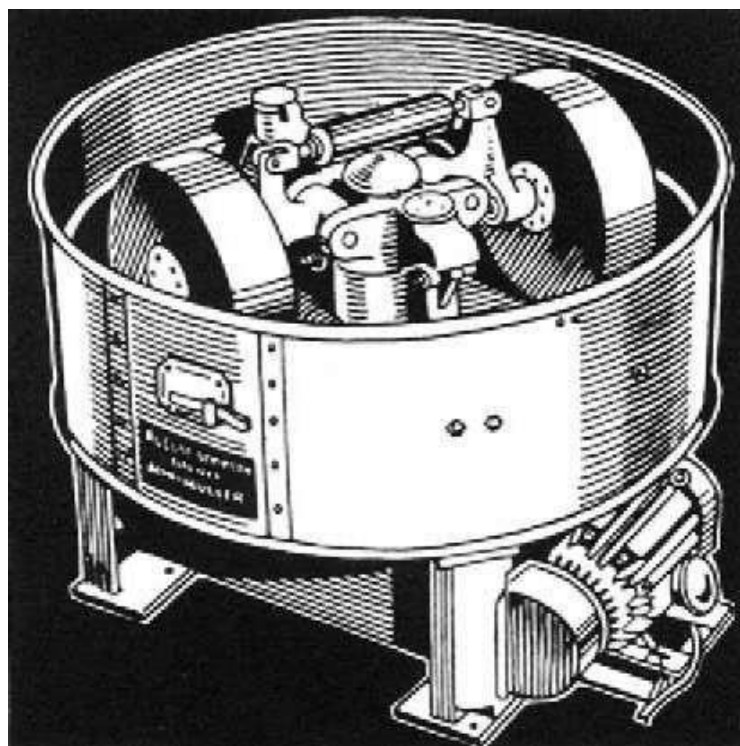
rasm. Qolip va o‘zak aralashmalaridan tayyorlaydigan beguni nomli aralashtirgich
