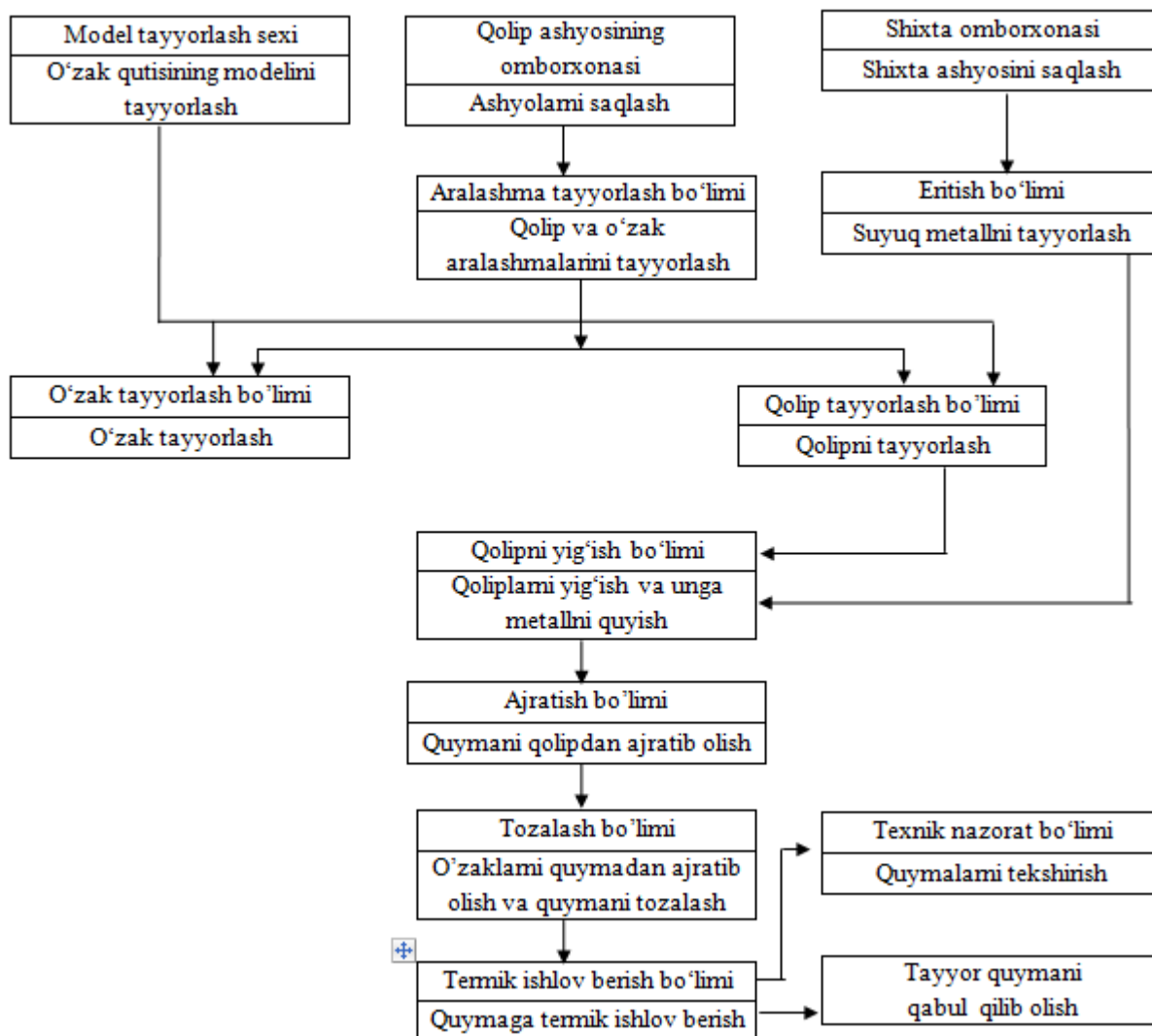
1-rasm. Quyma olishning texnologik sxemasi
