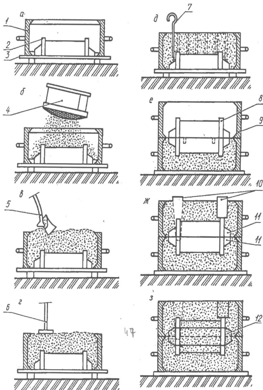
21-rasm. Vtulka quymasini qoliplashning texnologik jarayoni:
