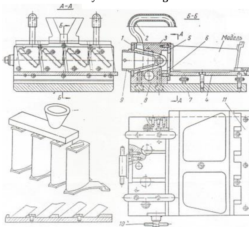
32-rasm. Kovsharlash yo'li bilan ulangan moslamalar bloki.
