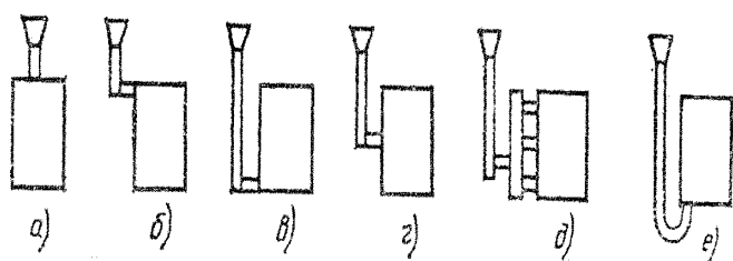
11-rasm. Turli usullarda suyuq metallni qolipga yetkazib beruvchi tizimlar
