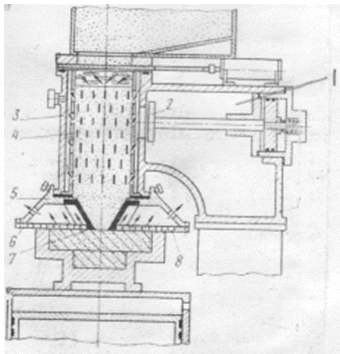
30-a rasm. Qumotar mashinada o'zakni tayyorlash sxemasi
