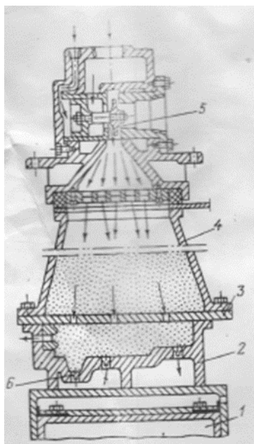
30-rasm. Qum puflash mashinasi sxemasi:
