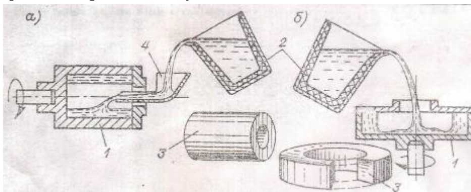
37-rasm. Markazdan qochma kuch yordamida quyma olish sxemasi.
