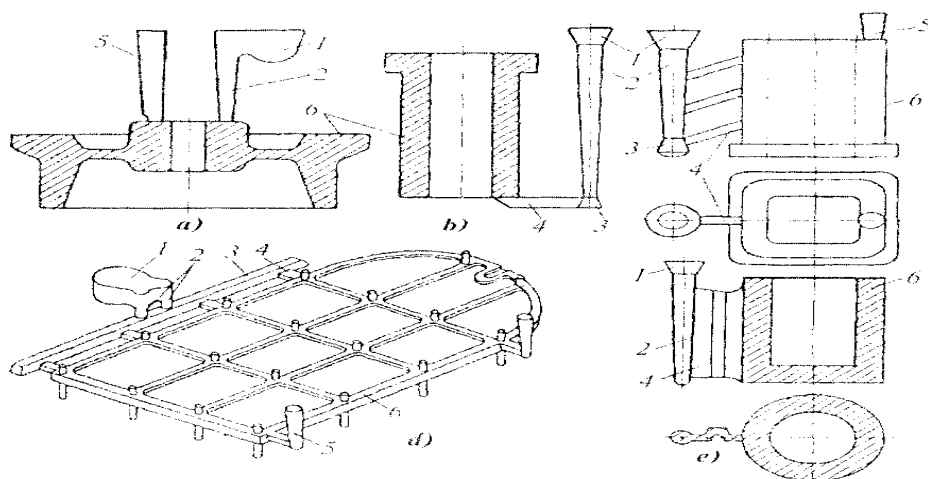
12-rasm. Quyish tizimining turlari:
