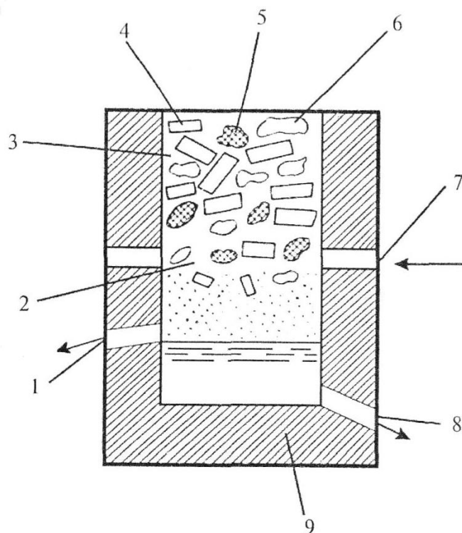
43-rasm. Metallarni suyuqlantirish pechining umumiy tuzilishi:
