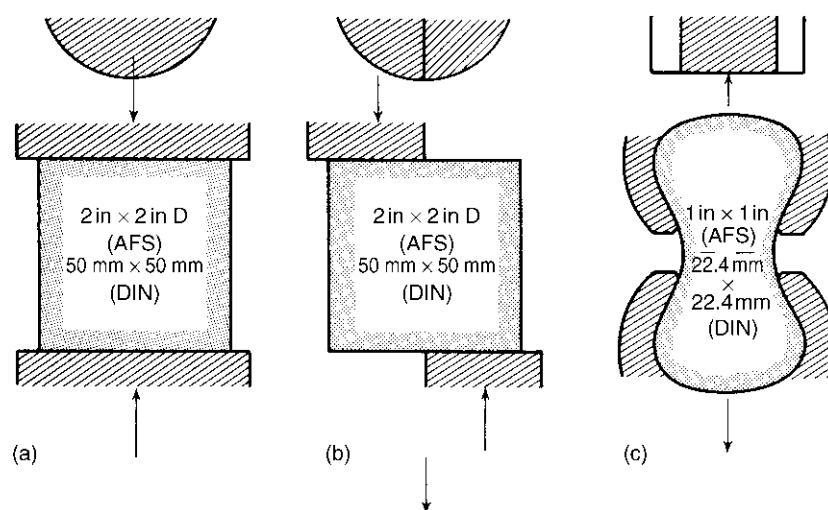
rasm. Qolip va o‘zak aralashmalaridan namunalarni sinash usullari
