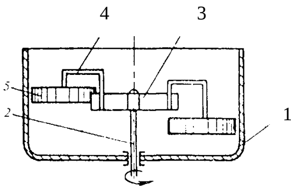
8.4 – rasm. Gorizontal joylashgan g‘ildirakli aralashtirish yugurdaklari.
