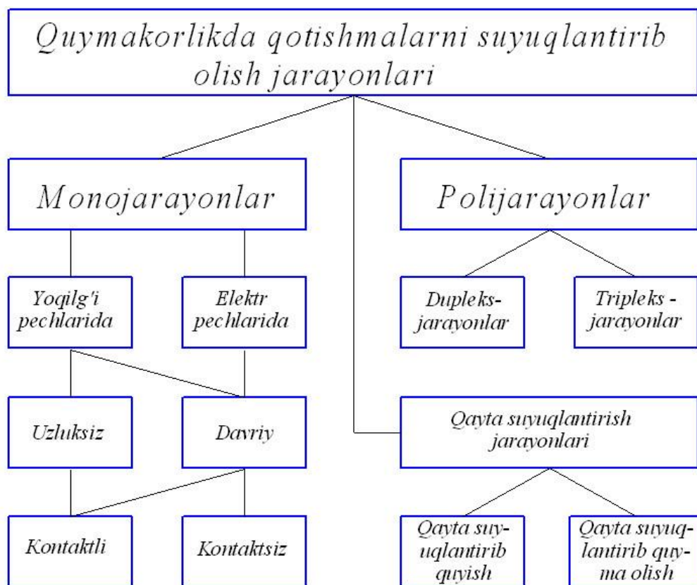
44-rasm. Quymakorlikda qotishmalarni suyuqlantirib olish jarayonlarining klassifikatsiyasi.
