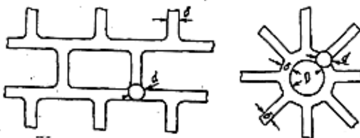
48-rasm. Bo'rtmalarning detallarda bajarilish variantlari
