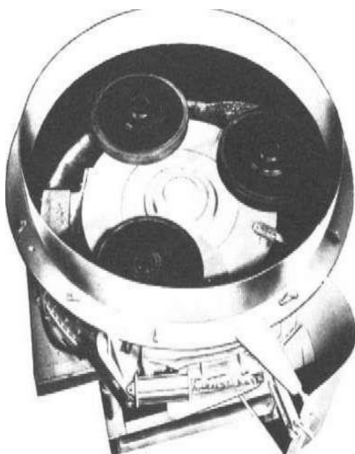
rasm. Tezligi yuqori bo'lgan qolip aralashmalasini tayyorlash jihozi
