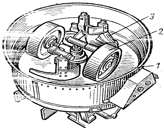
9 – rasm. Qolip aralashmasini tayyorlab beradigan qorishtirgich (begun):
