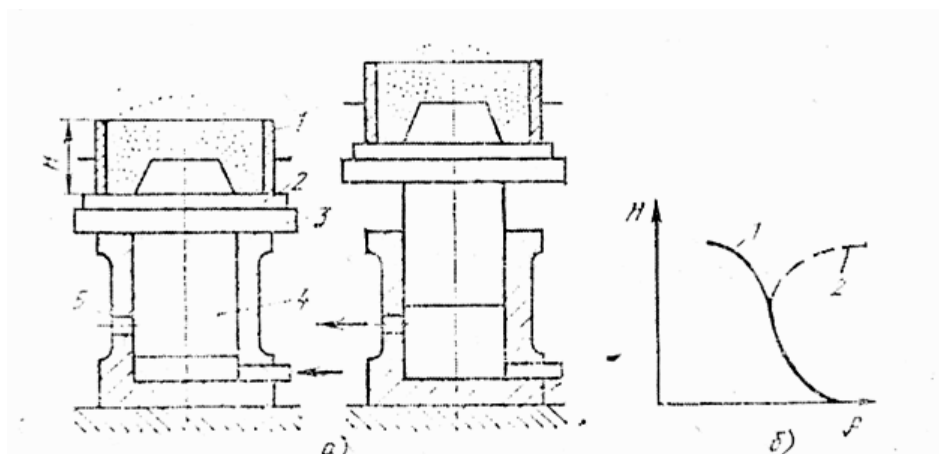
24 rasm. Silkitish qoliplash mashinasining ishlashi va opokaning balandligiga qarab zichligining taqsimlanishi:
