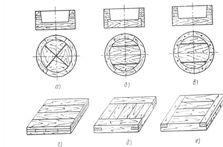
4-rasm. Puxtaligi bo'yicha 3 sinfga bo'lingan moslamalar:
