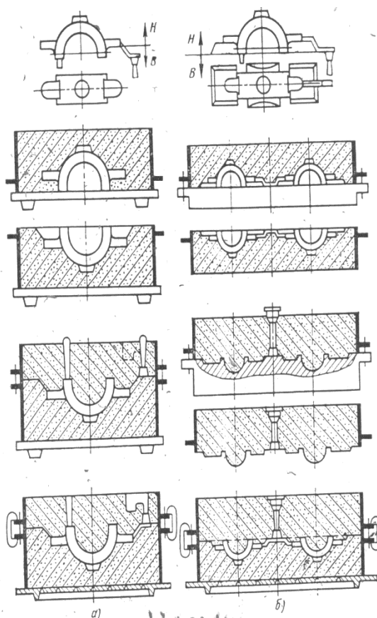
22-rasm. Podshipnik qopqog‘ini qo‘lda (a) va mashinada tayyorlash (b) sxemasi
