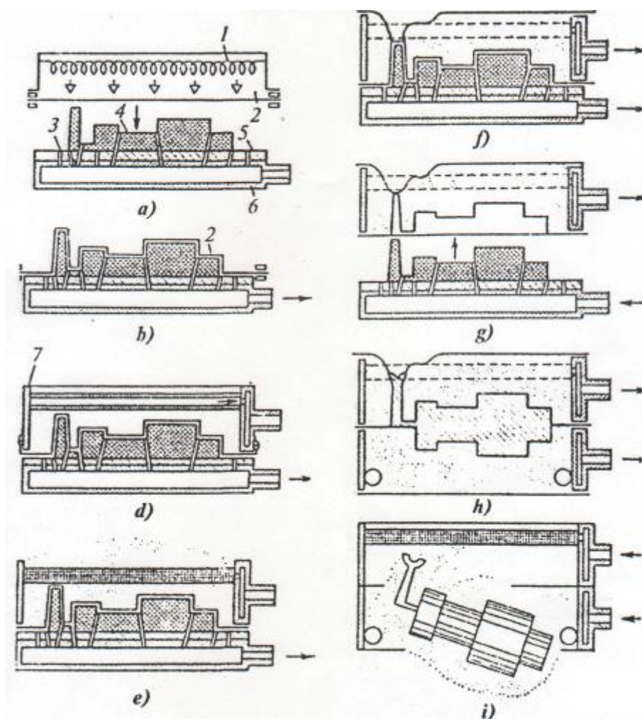
27-rasm. Vakuum yordamida qoliplash chizmasi:
