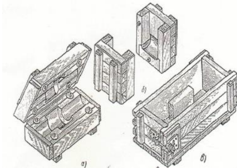
28- rasm. Yog'ochdan ishlab chiqilgan o'zak qutilari:
