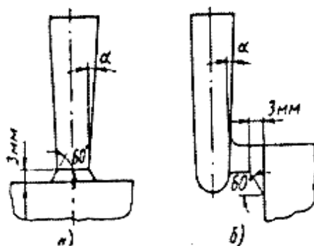
18-rasm. Xovuraklar: a-to'g'ri; b-chetlatuvchi
