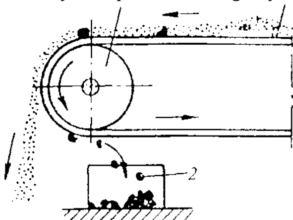
7-rasm. Magnit separatorining chizmasi.
