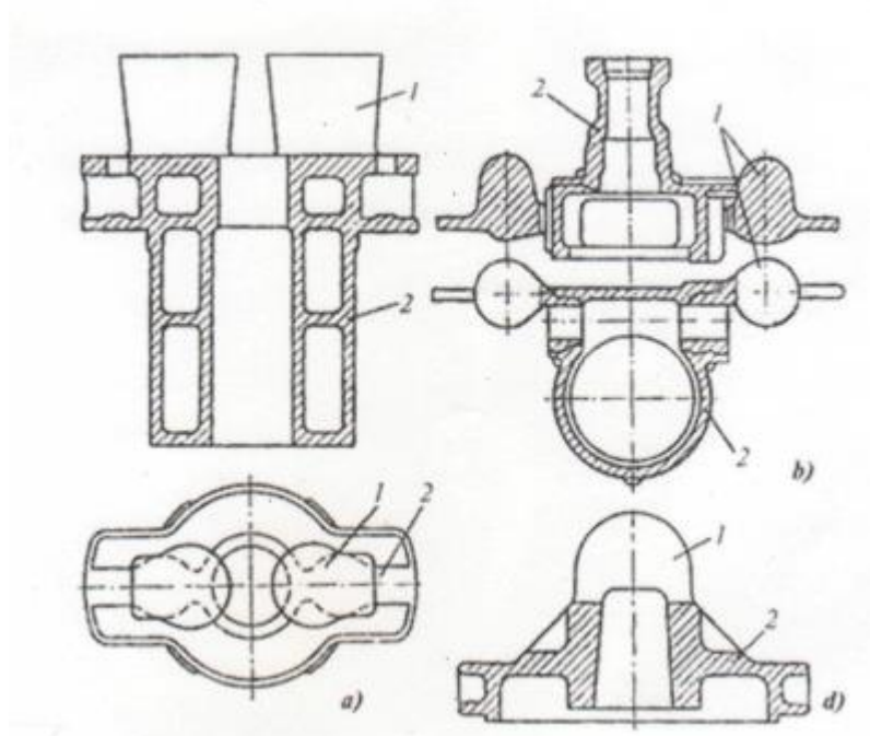
49-rasm. Ustama ta'minlagichlarning turlari:
