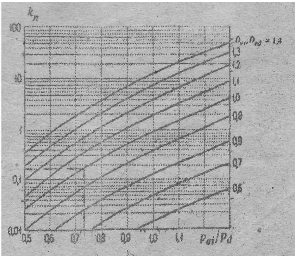
1-rasm. Qattiq bo'lmagan qoplamalar uchun og'irlikni hisobiya keltirish uchun koeffitsient K_n ni aniqlash uchun nomogramma.
