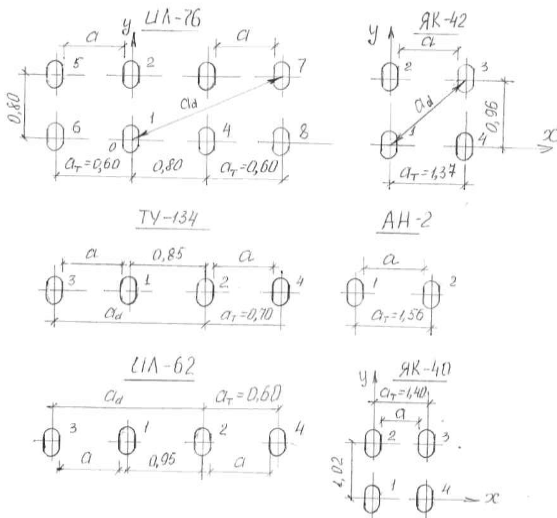
2-rasm. Qattiq va qattiq bo'lmagan aerodrom qoplamalari uchun ekivalent yakka g'ildirakli og'irlikni aniqlash sxemasi: I-YI tayanchning hisobiysxemalari(davomi).
