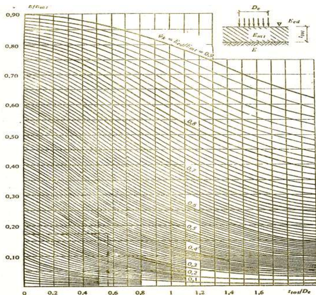
3-rasm. Qattiq bo'lmagan qoplama uchun \psi_{\kappa} koeffitsientni aniqlash uchun nomogramma.
