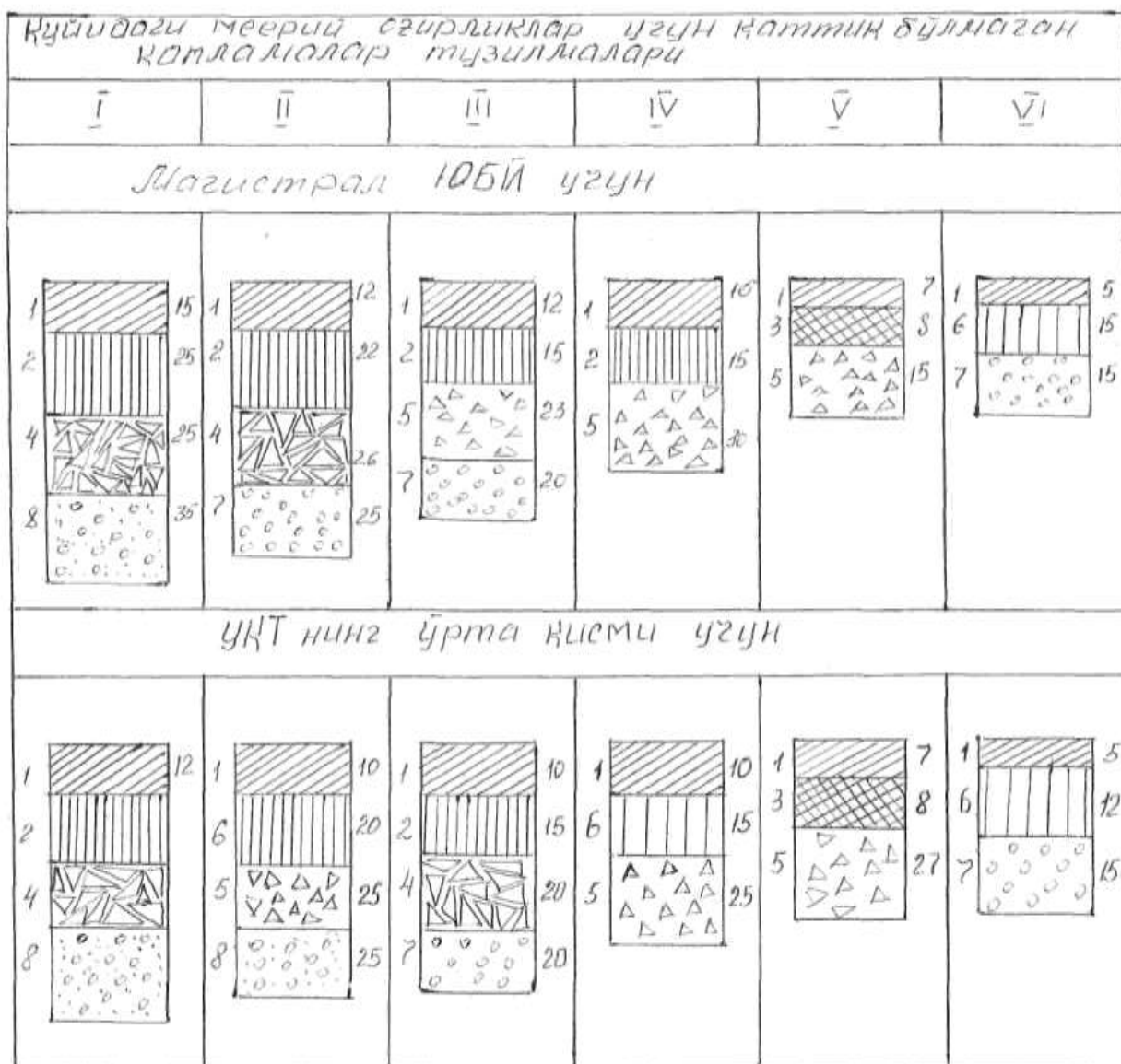
2-рasm. Турли ме'йорий og'irlik darajalari uchun qattiq bo'lmagan aerodrom qoplamalarining tavsiya etiladigan tuzilishi(o'ng tomondagi raqamlar qatlam qalinligini ko'rsatadi, santimetrda).
