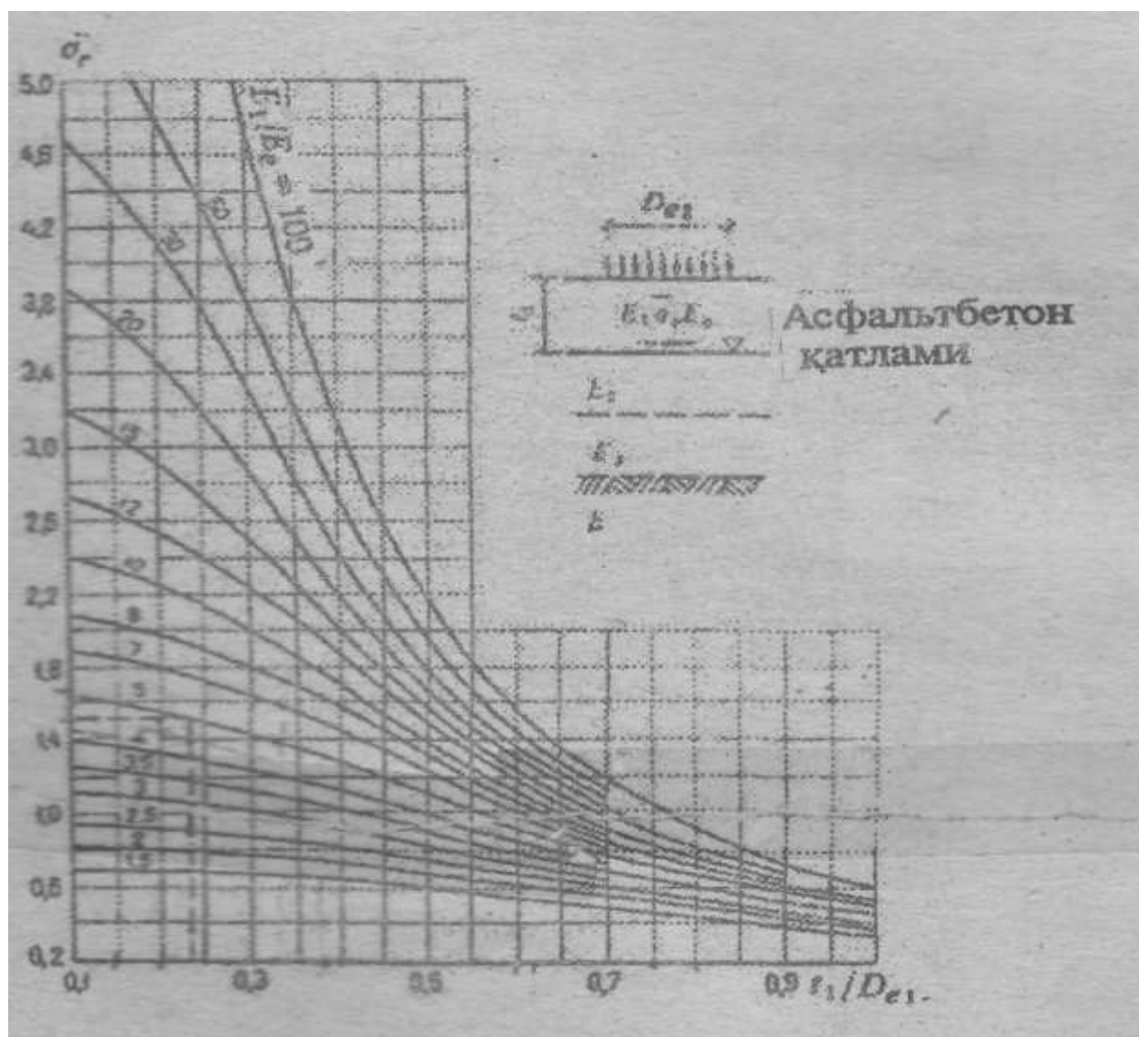
5-rasm. Og'irlikdan asfaltbetonda yuzaga keladigan solishtirma cho'zuvchi kuchlanish \bar{\sigma}_r ni aniqlash uchun nomogramma.
