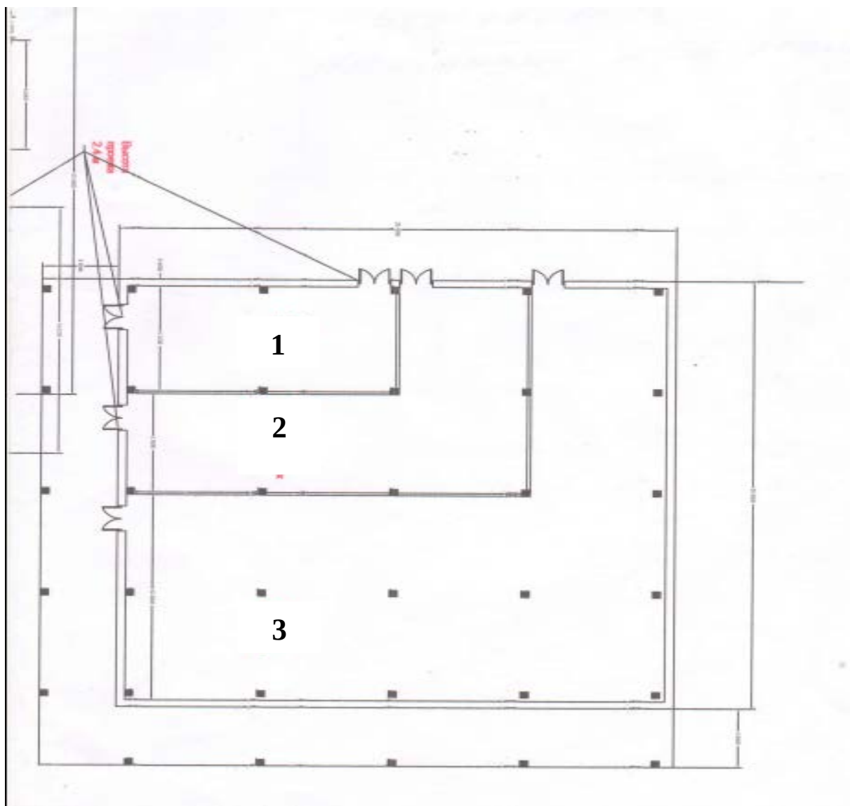
25-расм. Омборхона лойиҳаси:
