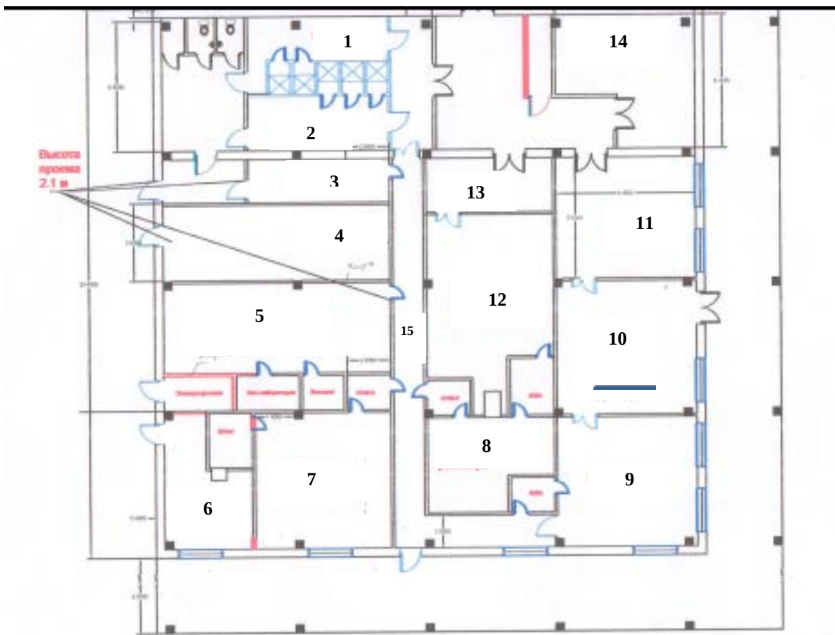
24-расм. Ишлаб чиқариш биноси лойиҳаси:
