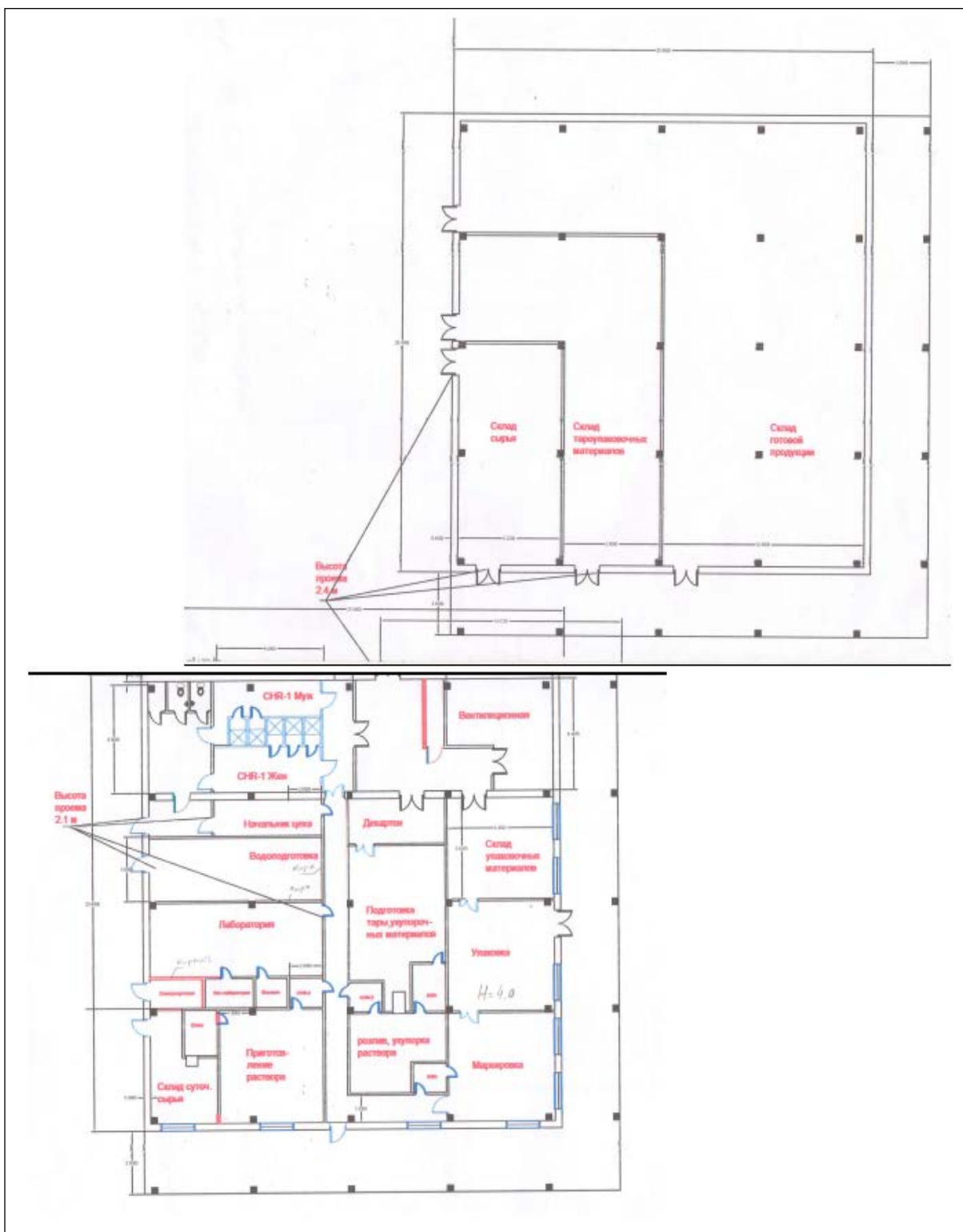
23-расм. Ишлаб чиқариш ва омбор биноси умумий лойиҳаси.
