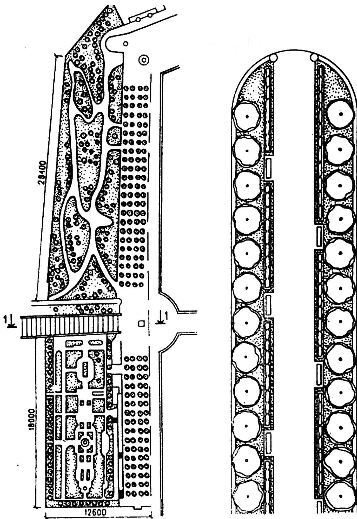
113-расм. Хиёбонларнинг меъморий чизмаси
