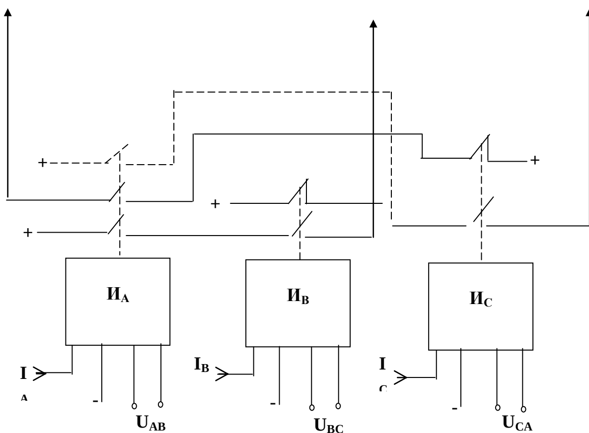
16-rasm. Ishga tushiruvchi qarshilik relesining o'zaro siklik bloklangan sxemasi.
