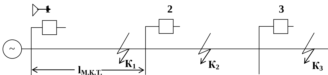
2-rasm. Masofali himoyaning sabr vaqtini qisqa tutashuv nuqtasigacha bo'lgan l_{M.Q.T.} ga bog'liqligi.
