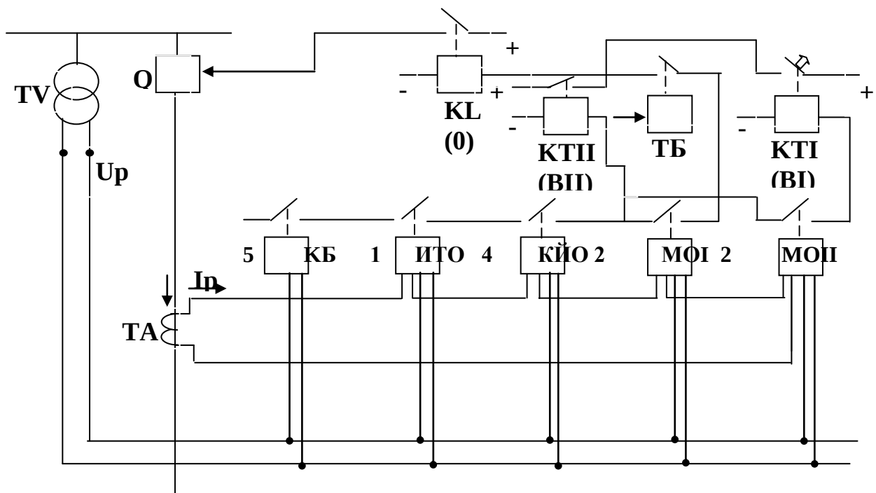
7-rasm. Uch pogʻonali masofali himoyaning soddalashtirilgan sxemasi.
