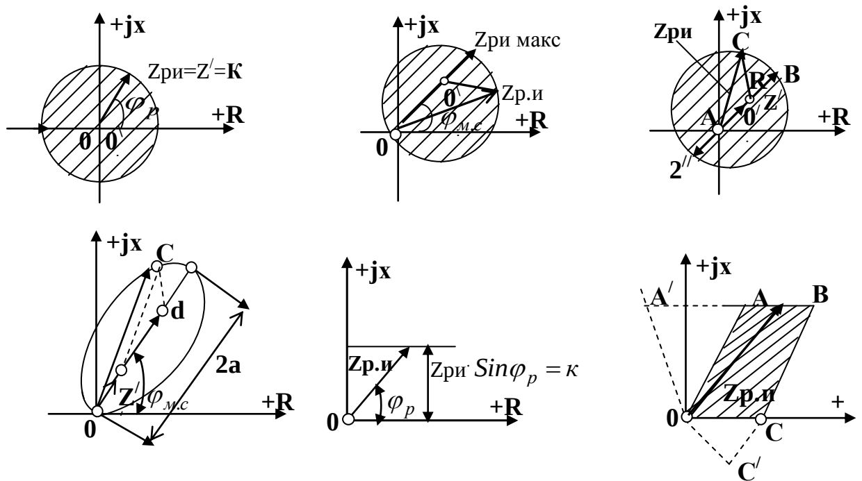
9-rasm. Qarshilik relesini ishlash tavsiflari.
