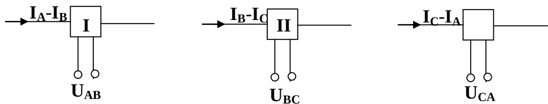
10-rasm Masofa organlarini ulanish sxemasi.
