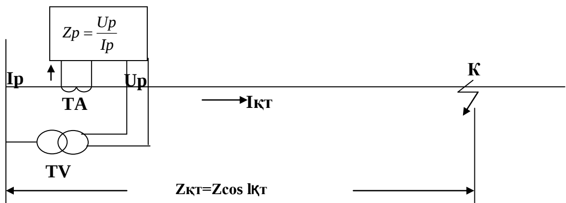
10-rasm Masofa organlarini ulanish sxemasi.
