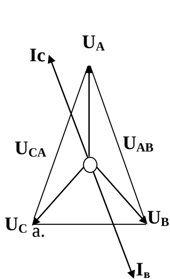
12-rasm. BC fazalarda ikki fazali qisqa tutashuvda himoya o'rnatilgan joydagi tok va kuchlanishning vektordiagrammasi.
