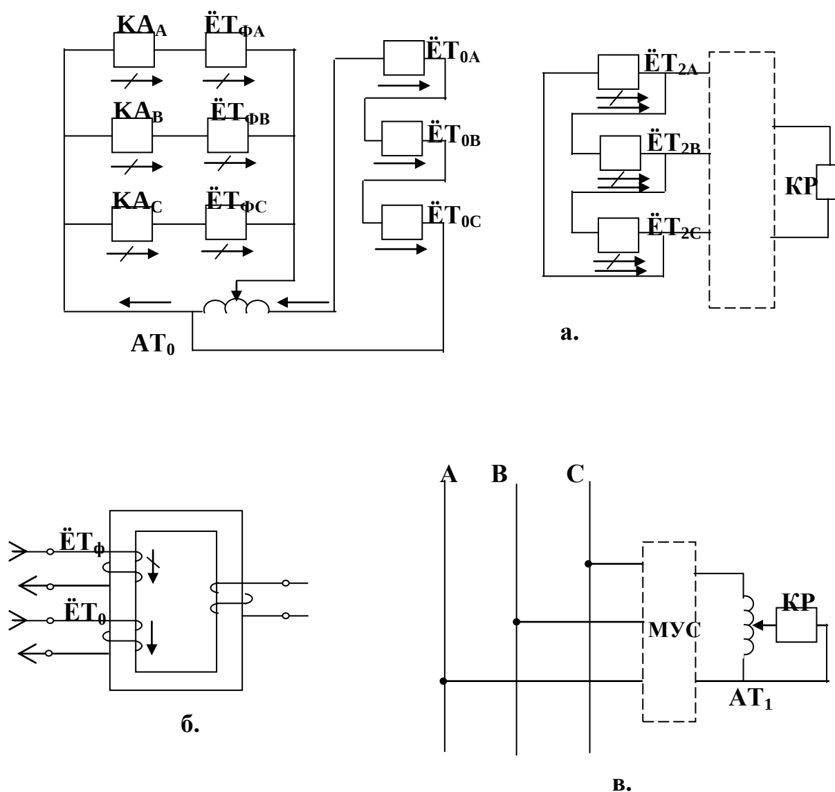
17-rasm. Bir masofa organli (qarshilik releli) bir sistemali soddalashtirilgan sxemasi.
