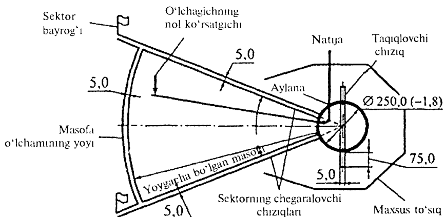
9-rasm. Disk uloqtirish joyi (o'lchamlar sm larda).
