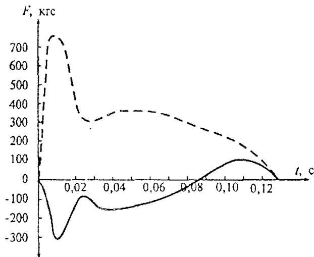
51-rasm. Yugurib kelib uzunlikka sakrashda depsinish dinamogrammasi (vertikal va gorizontali holati).
