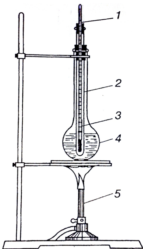
1-rasm. Suyuqlanish haroratini o'lchashga mo'ljallangan qurilma.
