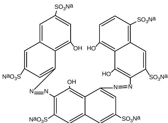
Kalsion (erioxrom qora) sulfarsazen
