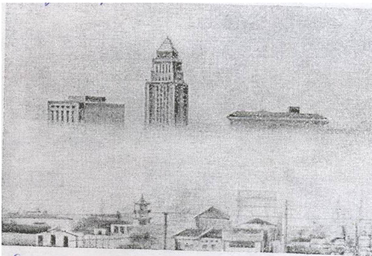
6-расм. Смог-захарли тутун аралаш туман (Лос-Анжелос)
