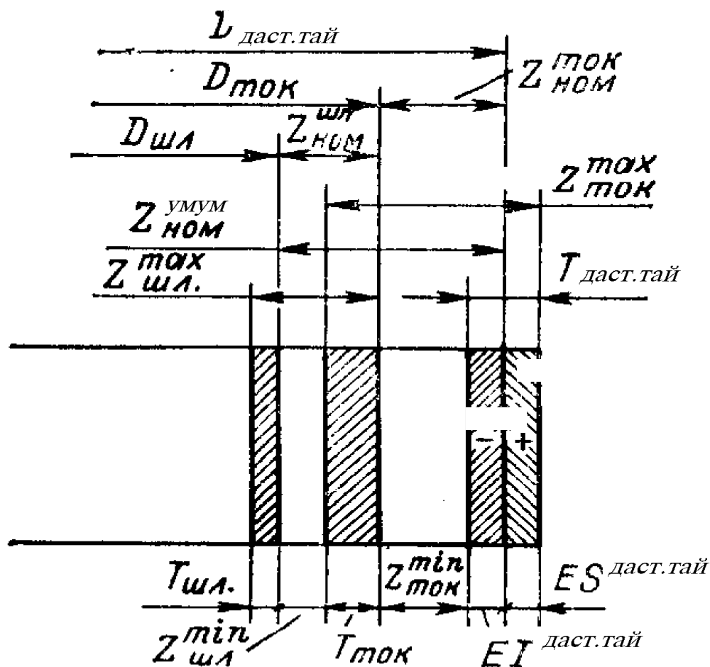
6.1-расм. Валга йўниш ва жилвирлаш орқали ишлов беришда қўйимларнинг ва допускларнинг жойлашиши
