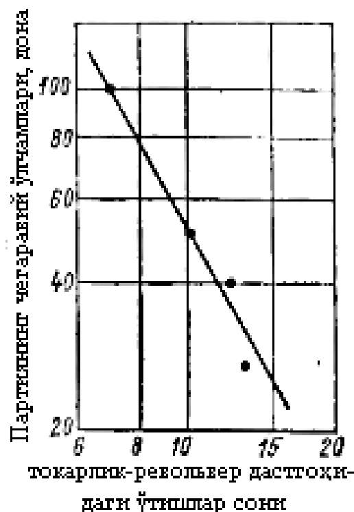
7.4-rasm. Zagotovkalarga ishlov berishni tokarlik-revolver dastgohidan bir shpindelli avtomatga oʻtkazishni iqtisodiy samaradorligi chegaralari grafigi
