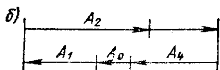
4.3-рasm. Ўлчам занжирларини куриш
