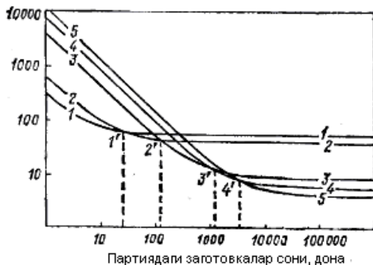
7.3 rasm. Pog'onali vtulkalarni turli jihozlarda tayyorlashda tannarxning o'zgarishi:
