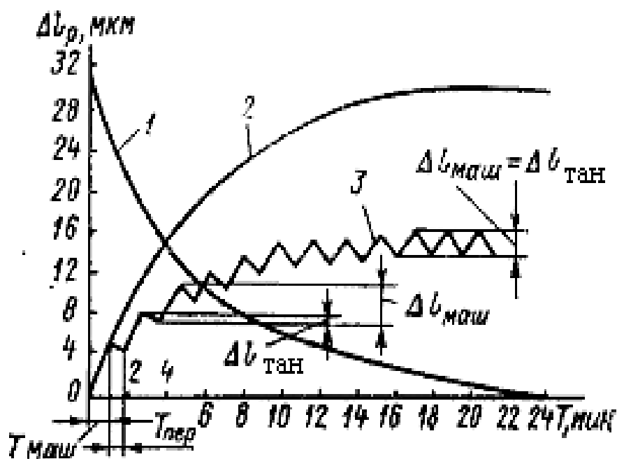
2.5-rasm. Keskichning tanaffus bilan ishlashida қизишдан унинг деформацияланишига таъсири:
