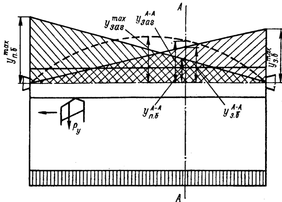
3.1-расм. Технологик тизимнинг эластик қайтиши
