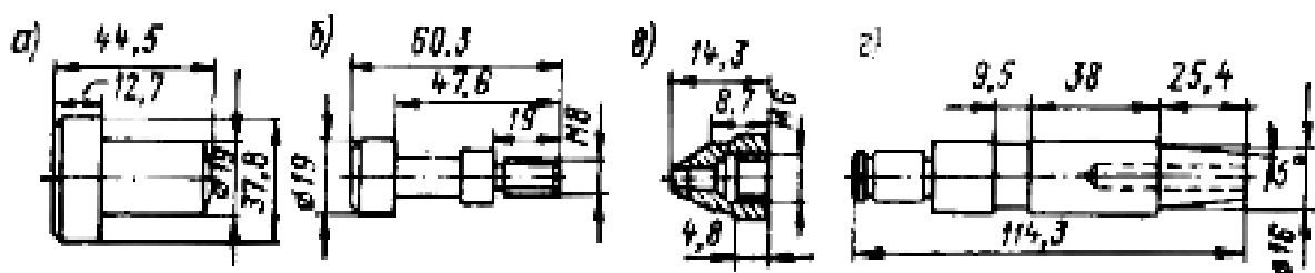
7.5-rasm. Tokarlik-revolver dastgohlari va avtomatlarda ishlov beriladigan tipik zagotovkalar
