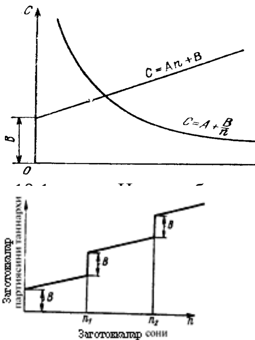
10.2-расм. Қўшимча жиҳоз қўллаш натижасида тannарх C нинг ўзгариши
