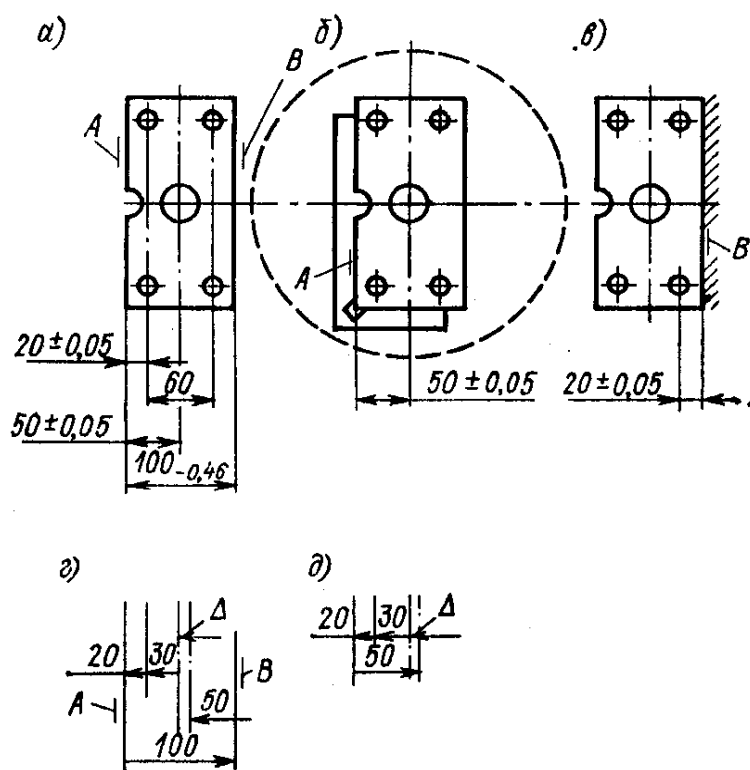
5.8-расм. Пармалаш ва йўниб кенгайтиришда базаларнинг доимийлик тамойилини
