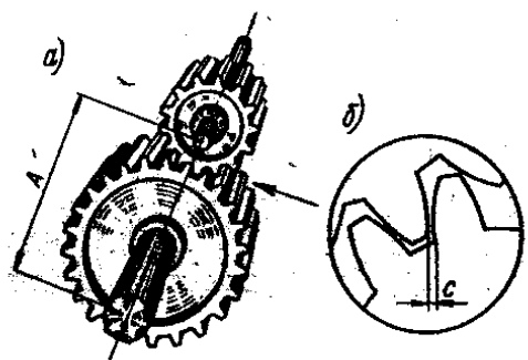
17.8-расм. Эволвентли тишли жуфтликни йиғишни текшириш
