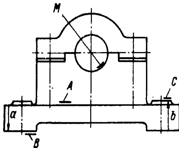
5.5-расм. Подшипник корпусига ишлов беришда дастлабки (дағал) ба- за
