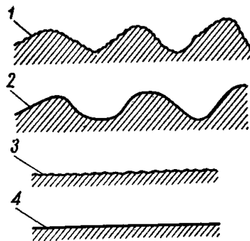
3.1-rasm. Yuzalarning turlari: 1- to'liqinsimon va g'adir-budir; 2-to'liqinsimon va toza; 3 – tekis va g'adir-budir; 4 - tekis va toza
