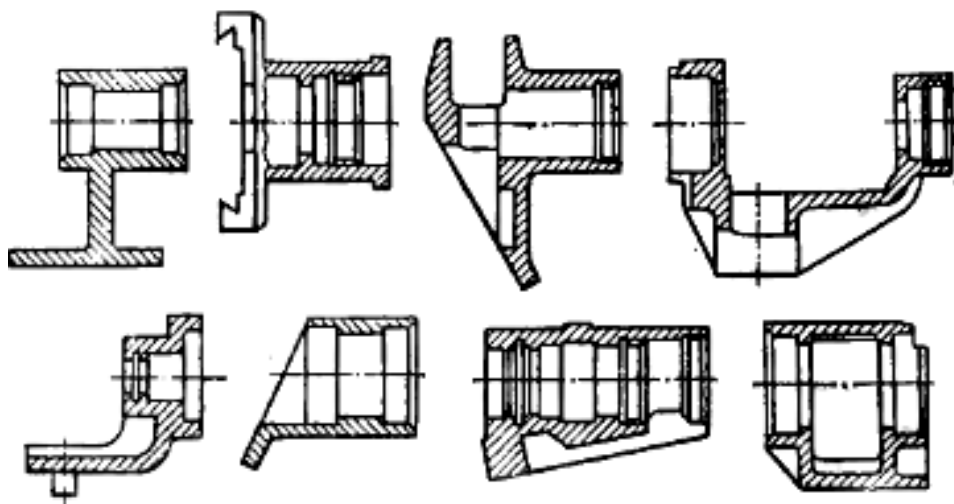
7.6-rasm. Bir marta sozlash bilan ishlov beriladigan zagotovkalar guruxi
