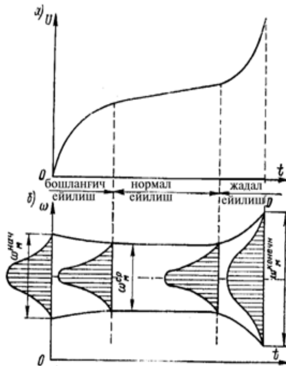
2.12-rasm. Kesuvchi asbobning eyilishi (a) va ishlov berilgan zagotovkalar o'lchamlarining oniy yoyilish maydonining o'zgarishi (b)
