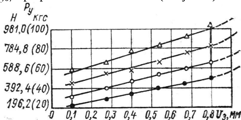
3.3-rasm. 2X13 markali po‘latni yo‘nishda kesish kuchi R_y ning keskichning orqa sirti eyilish maydonining kengligi E_m ga bog‘liqligi
