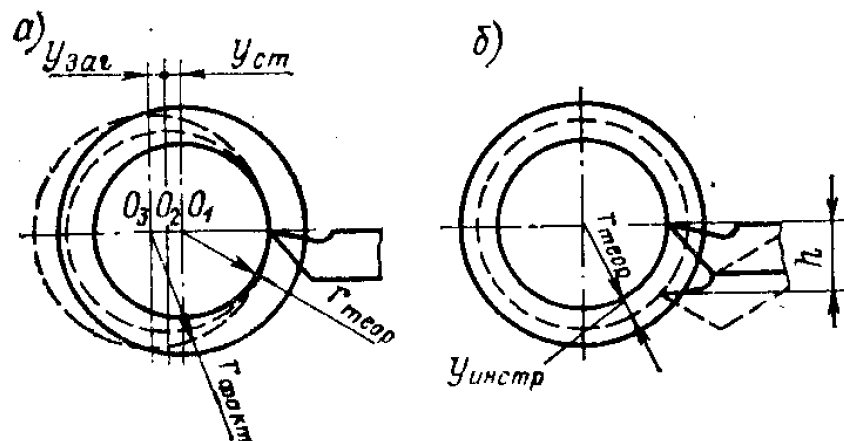
3.2-расм. Ишлов берилаётган заготловканинг ўлчамларига эластик силжишнинг таъсири:
