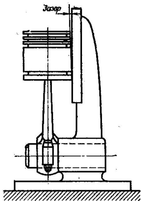
14.1-расм. Шатунни поршен билан йиғишни назорат қилиш мосламаси
