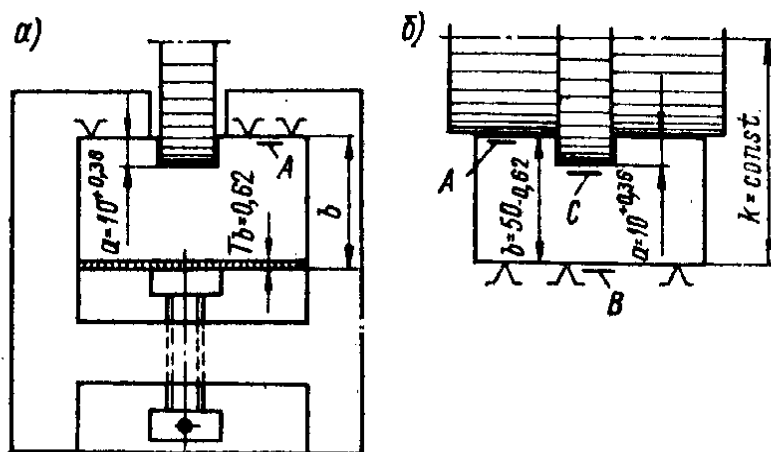
5.7-рasm. Конструкторлик база билан мос тушган технологик база A бўйича пазни фрезалаш
