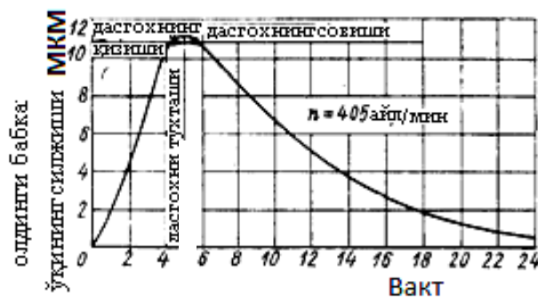
2.4-расм. Токарлик дастгоҳининг марказларида ишлов беришда олдинги бабканинг қизиши натижасида унинг ўқининг горизонтал йўналиш бўйича силжishi олдинги бабка:
