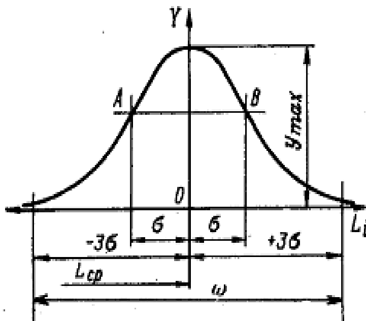
2.9-расм. Ўлчамлар ёйилиш майдонининг ўртаси \omega га нисбатан тақсимланиш эгри чизиғи чўққисининг силжиши
