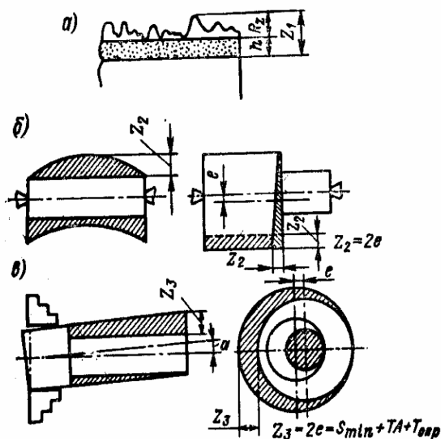
6.2-рasm. Операцион кўйим элементларининг таркиби
