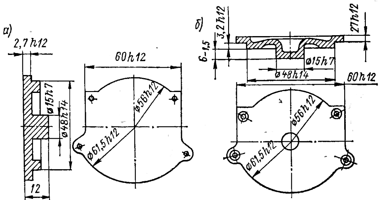
10.1-rasm. Tutqich qopqog'i konstruksiyasi
