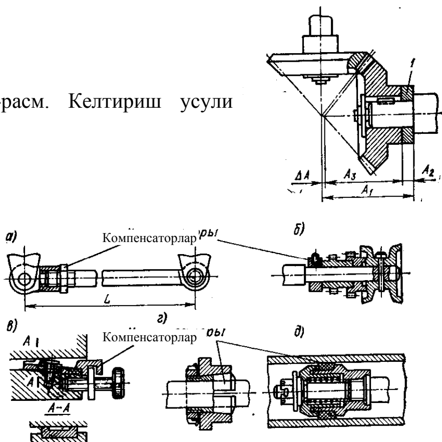
13.3-rasm. Qo'zg'aluvchan kompensatorni qo'llash orqali yig'ish
