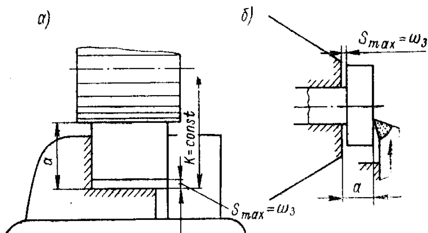
2.14-рasm. Фрезалаш (a) ва токарлик ишлов беришда (б) маҳкамлаш хатолиги
