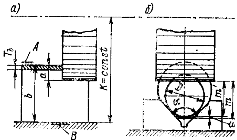
2.13-рasm Базалаш хатолиги \omega_{\Delta} = \omega_{\phi} нинг келиб чиқиши
