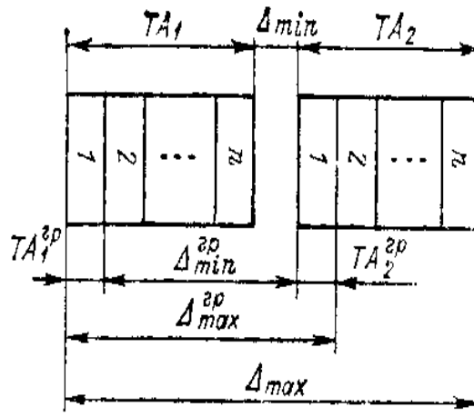
13.1-rasm. Guruhli dopuskni aniqlash sxemasi
