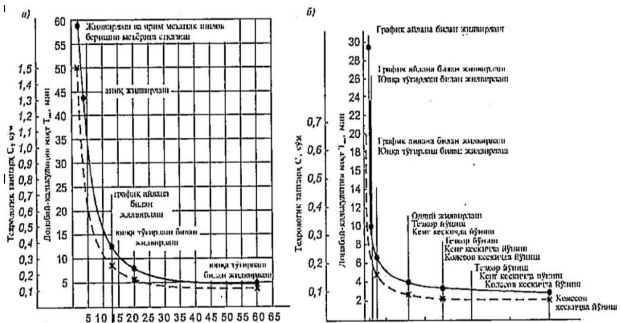
8.1-rasm Zagotovkalarga ishlov berish ish hajmi va tannarxining sirt aniqligi va g‘adir-budirligiga bog‘liqligi:
