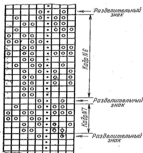
11.1-rasm. Dastur kadrlarini perfolentada joylashuvi
