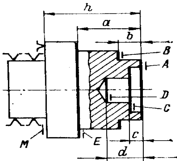
5.4-расм. Заготовка револьверли дастгоҳда ишлов беришда созлаш базаси А дан фойдаланиш
