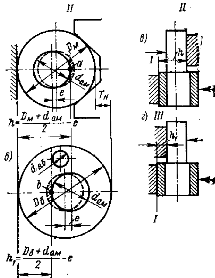
17.3-расм. Валик ва втулкани автоматик йиғишда бикр
