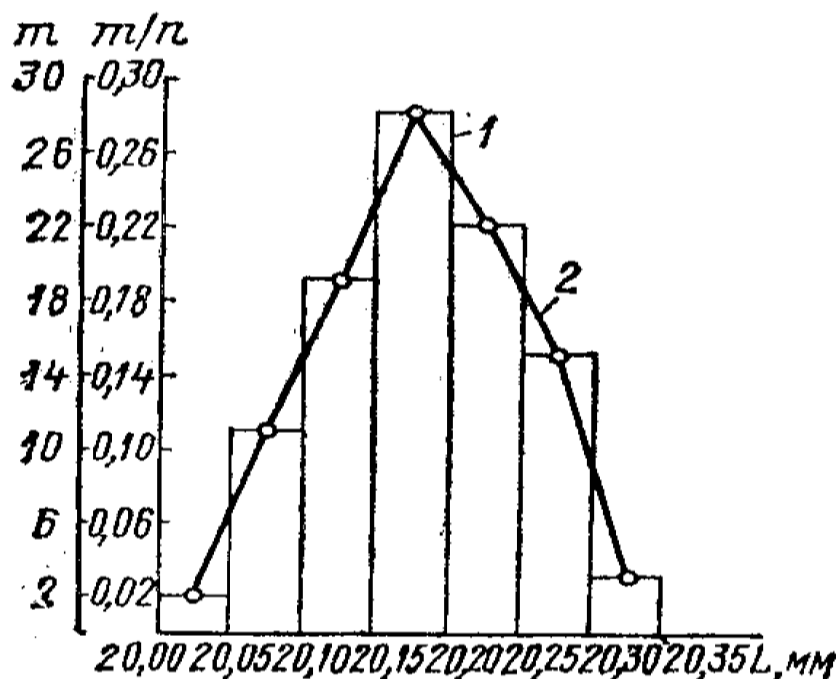
2.6-расм. Заготовкalar ўлчамларининг тақсимланиши
