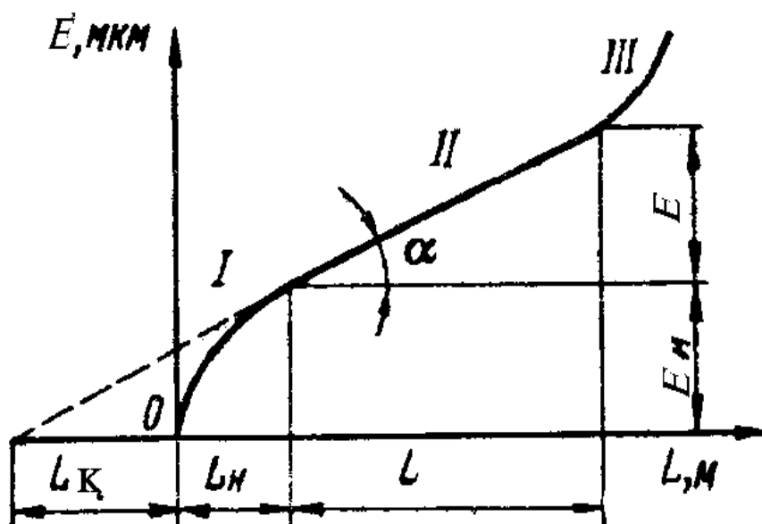
2.2-rasm. Kesuvchi asbobning yeyilishi E ni kesish yo'li uzunligiga bog'liqligi
