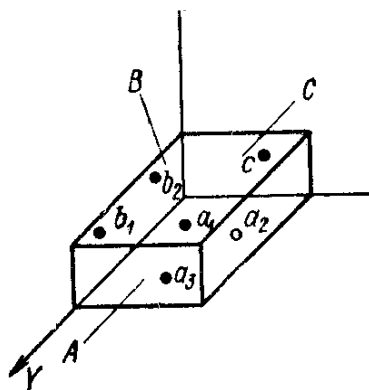
5.1-расм. Призма шаклидаги заготувкани мосламада базалаш
