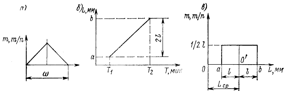
2.10-рasm. Ишлов беришда заготовкalar ўлчамларининг Симпсон (a) ва тенг эҳтимоллик қонунлари (б, в) бўйича тақсимланиши
