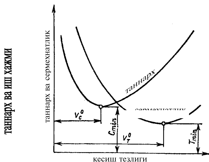
8.3-расм. Кесиш тезлигига ишлов бериш иш хажмининг ва таннархининг боғлиқлиги
