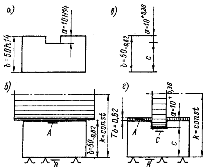
5.6-расм. Конструкторлик база билан мос тушмаган таянч технологик база B га нисбатан ариқчани фрезалаш
