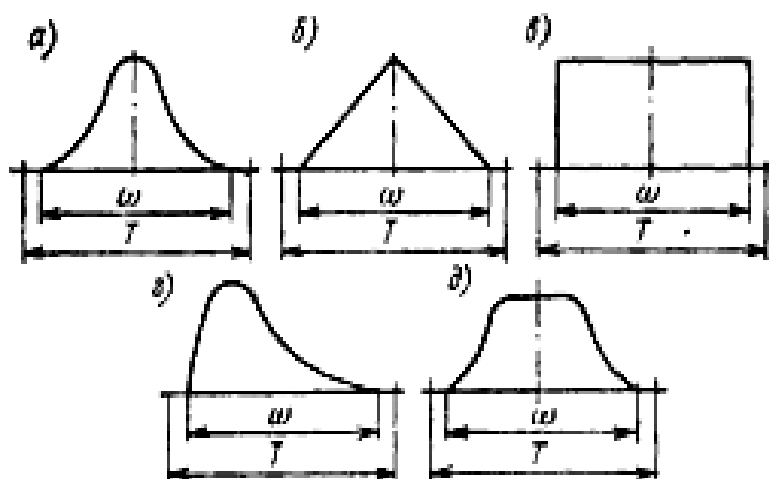
2.15-расм. Ўлчамларнинг турли тақсимланиш қонунлари учун заготовкаларга нуқсонсиз ишлов бериш шarti
