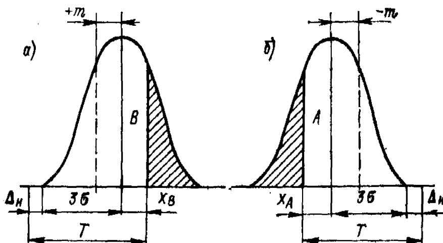
2.17-рasm. Тўғирлаш мумкин бўлган яроқсиз валларга (а) ва тешикларга (б) ишлов бериш учун дастгоҳларни созлаш
