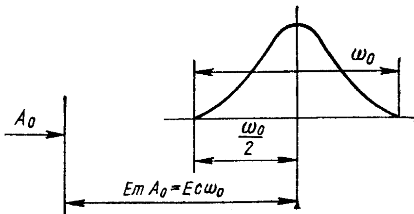
4.7-расм. Гаусс симметрик эгри чизиғи ёйилиш майдони ўртасининг координатаси E_c \omega_0 ва тўпланиш марказининг координатаси E_m A_0
