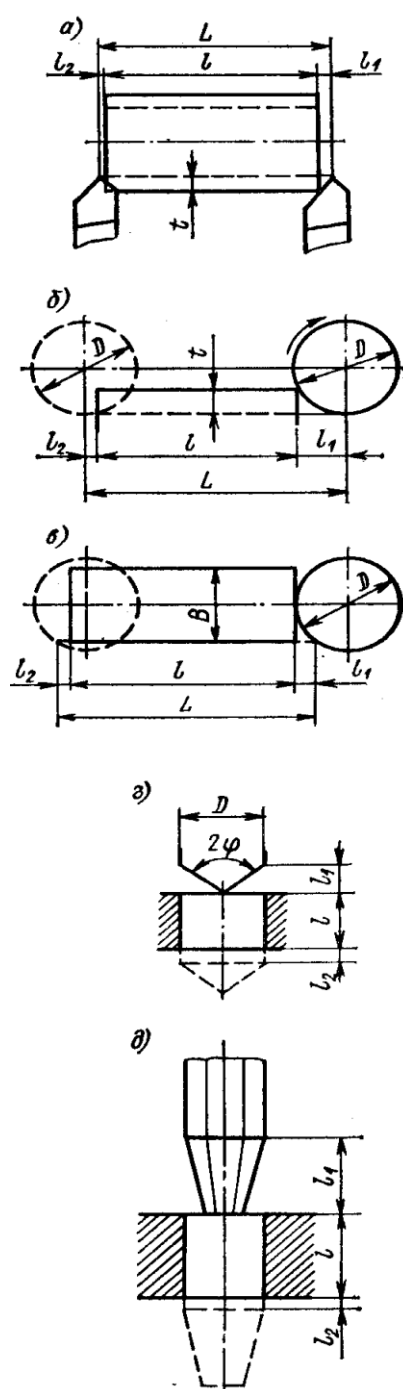
8.4-расм. Кесувчи ас- бобнинг юриш йўли:
