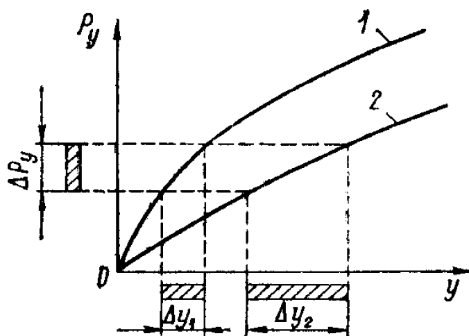
3.5-расм. Технологик тизим бикрлигининг эластик силжишнинг тебраниши \Delta y_1 ва \Delta y_2 га таъсири.
