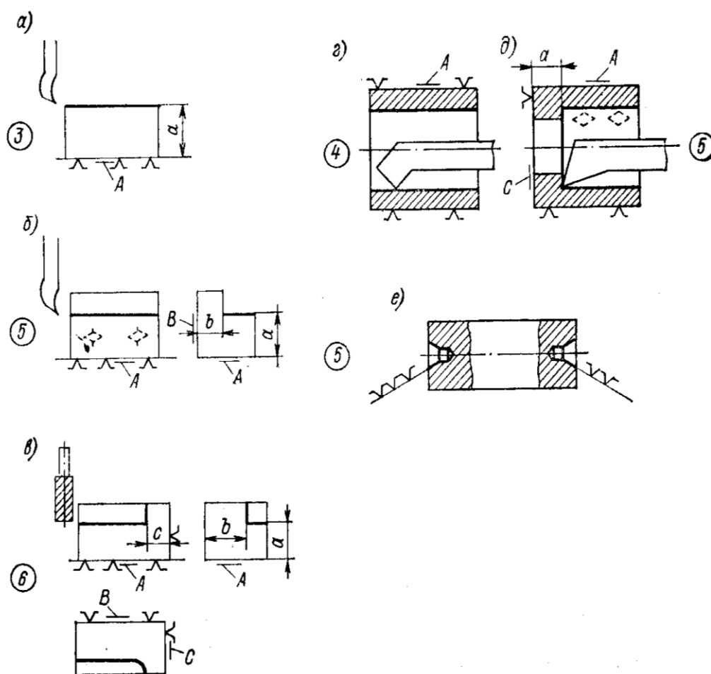
5.3-расм. Заготовкам ишлов беришда битта (а, с), иккита (б, д, е) ва учта (в) базалардан фойдаланиш
