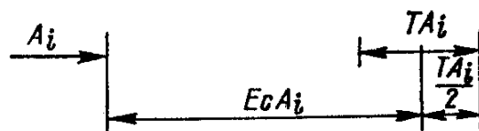
4.4-рasm. Допуск майдони TA_i ўртасининг координатаси E_c A_i
