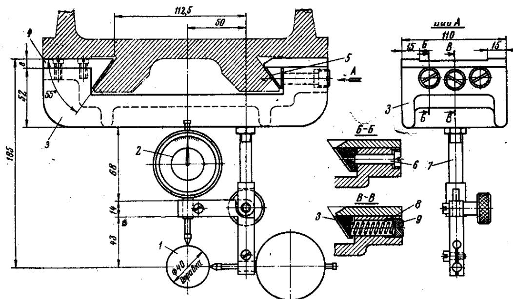
14.2-расм. Консолли фрезалаш дастгоҳи хартуми ҳолатининг шпиндель ўқиға нисбатан паралеллигини назорат қилиш мосламаси
