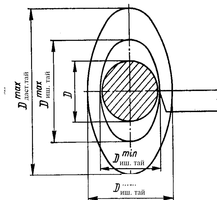
3.4-расм. Дастлабки заготровка шакл хатоликларининг ишлов берилган деталларнинг шакл хатоликларига таъсири
