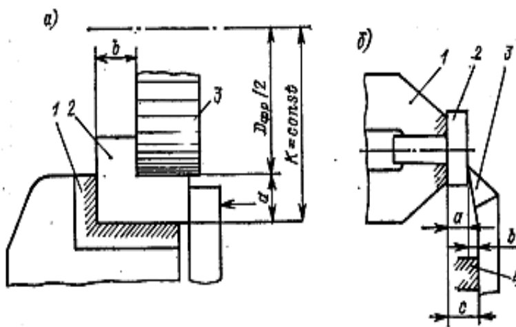
2.1-rasm. Zagotovkalarga ishlov berishda o'lchamlarni avtomatik olish usuli
