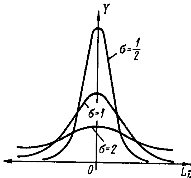
2.8-расм. Ўлчамларнинг нормал тақсимланиш эгри чизиги шаклига ўртача квадратик четга чиқишнинг таъси-
