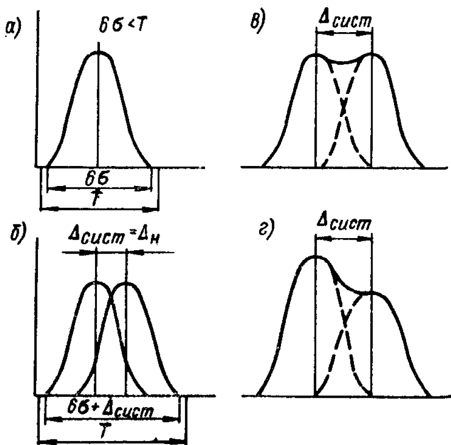
2.11-расм. Заготовкларнинг бир нечта партиясига дастгоҳни қайта созлаш билан ишлов беришда \Delta_{munt} таъсири натижасида тасодифий хатоликларнинг йиғинди эгри чизиги шаклининг ўзгариши
