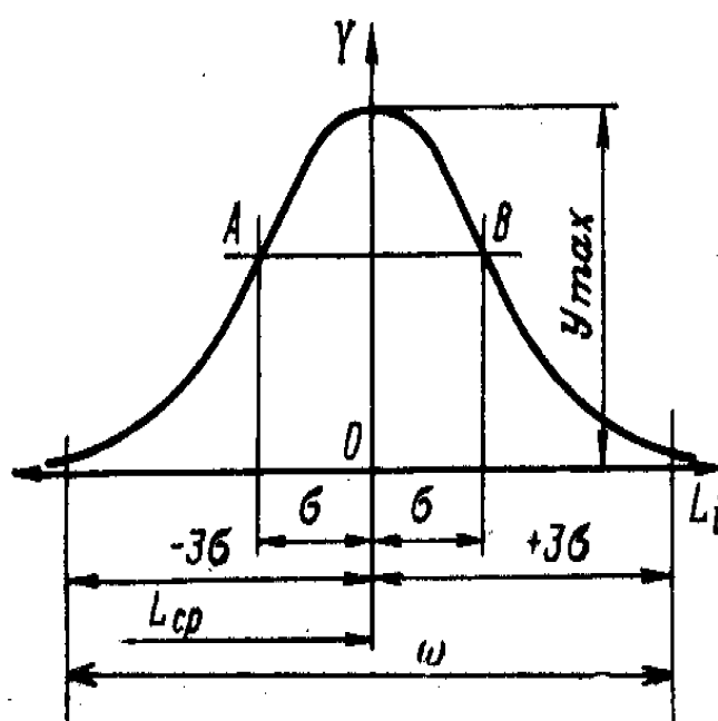
2.7-расм. Ўлчамлар нормал тақсимланишининг эгри чизиғи
