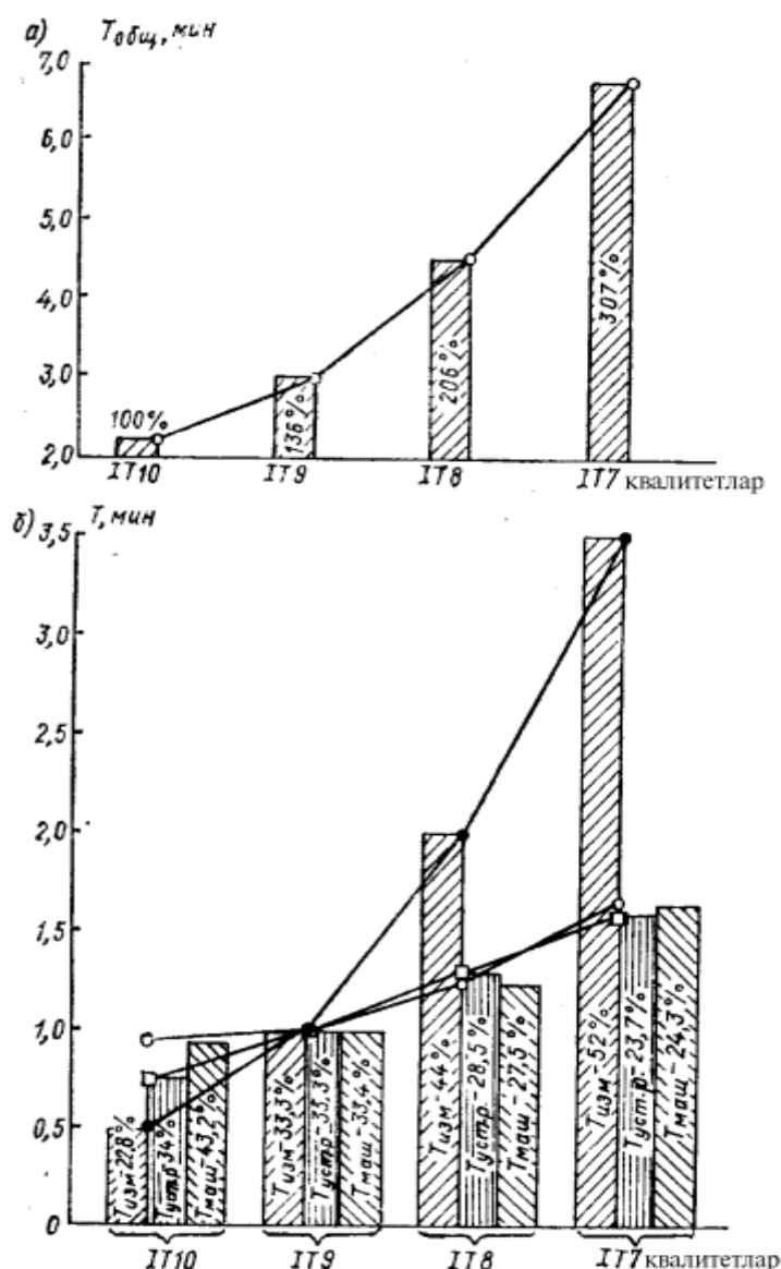
8.2-расм. Ишлов бериш иш хажмининг талаб қилинган аниқликка боғлиқлиги:
