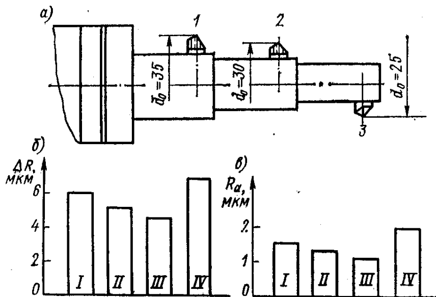
3.7-расм. 45 маркали пўлатдан тайёрланган заготовкада йўнилган тешикларнинг аниқлигига кўп кескичли ишлов беришнинг таъсири:
