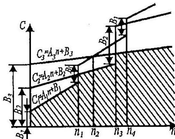
10.3-расм. Технологик жараёнларнинг учта таннархларини солиштириш (кам харажатли майдон штрихланган)
