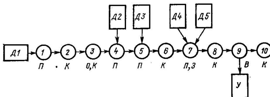
17.2-rasm. Uzelli avtomatik yig'ishning texnologik sxemasi
