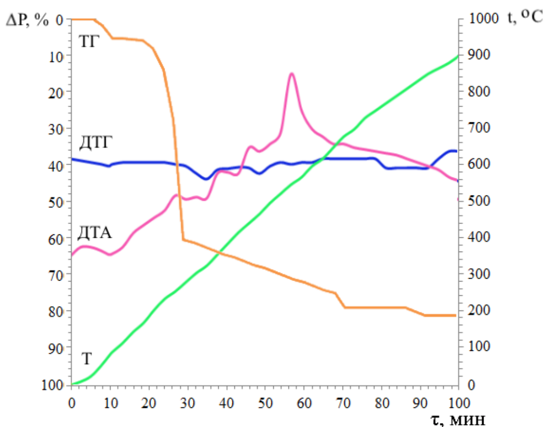
3.7-рasm. L 3 лигандининг дериватограммаси.
