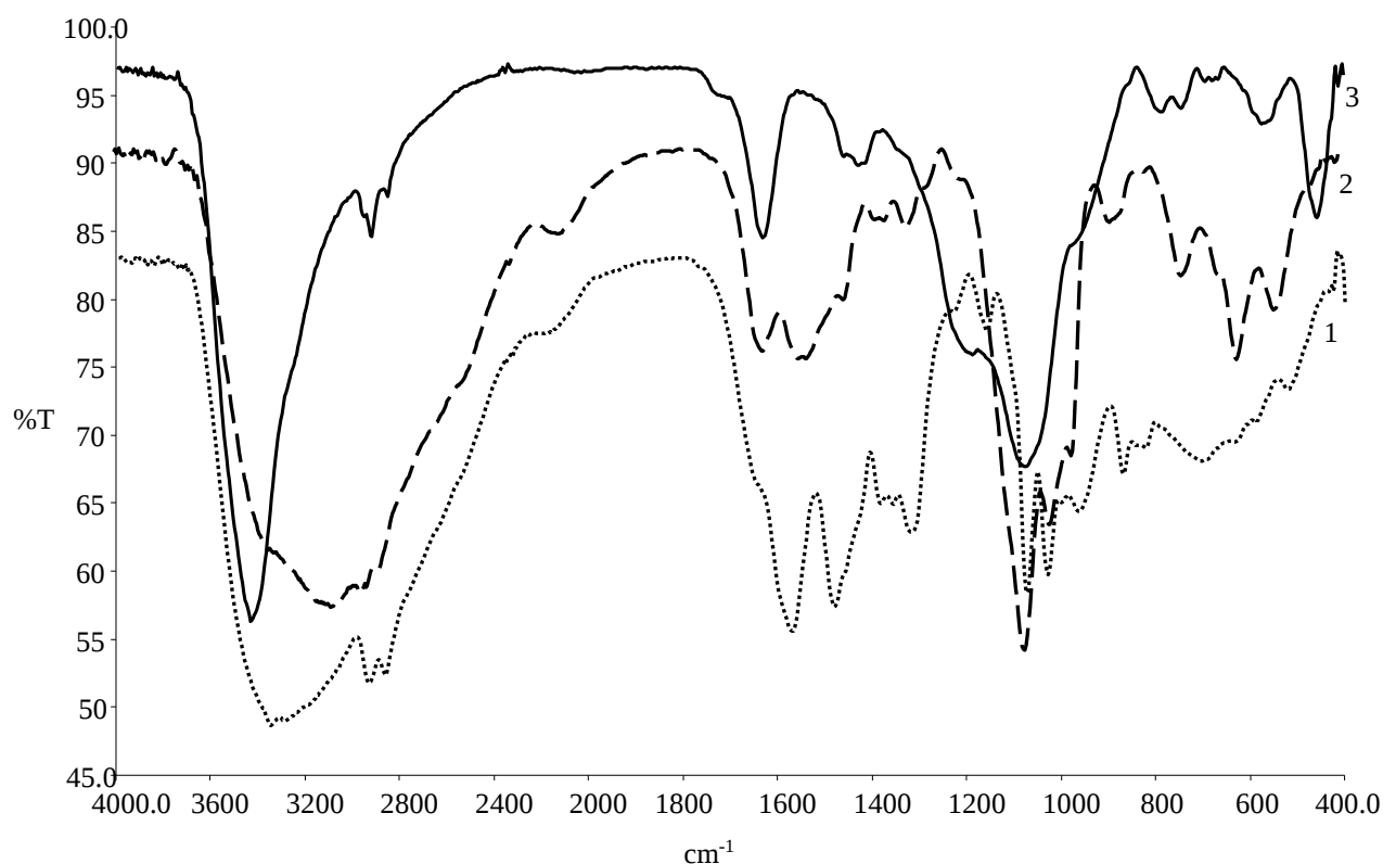
3.3-расм. Моноэтаноламин (1), калий О,О-ди-(2-аминоэтил)-дитиофосфат (2) ва улар асосида олинган лиганднинг (3) ИҚ-спектрлари.
