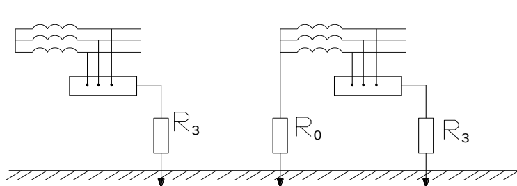
а-расм. Ерга улаш химояси схемаси
