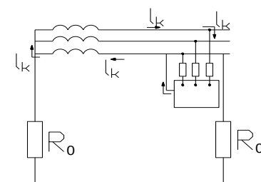
б-расм. Нолга улаш химояси схемаси.
