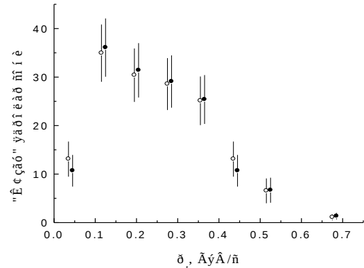
2-расм. {}^7\text{Li} (○) ва {}^7\text{Be} (●) “кўзгу” ядролар кўндаланг импульс тақсимоти
