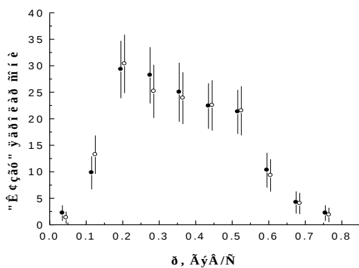
1-расм. Тинч ҳолатдаги кислород ядросида {}^7\text{Li} (○) ва {}^7\text{Be} (●) ядроси импульс тақсимоти
