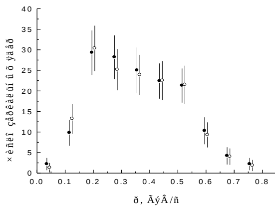
Рис. 1. Импульсные распределения ядер {}^7\text{Li} ( \circ ) и {}^7\text{Be} ( \bullet ) в системе покоя ядра кислорода
