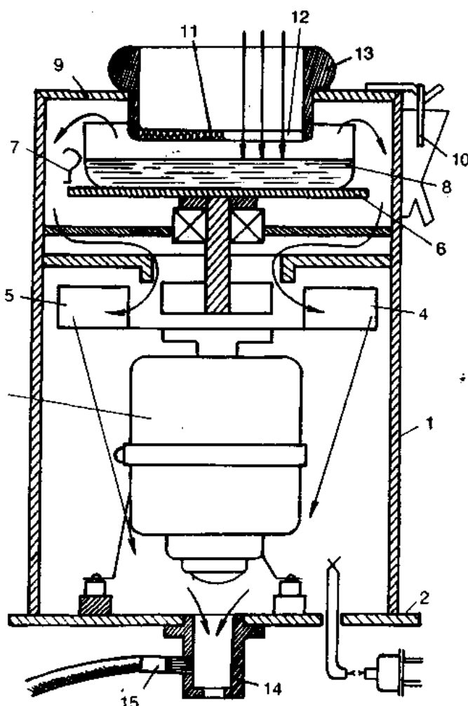
42-rasm. Krotov apparati (sxema).
