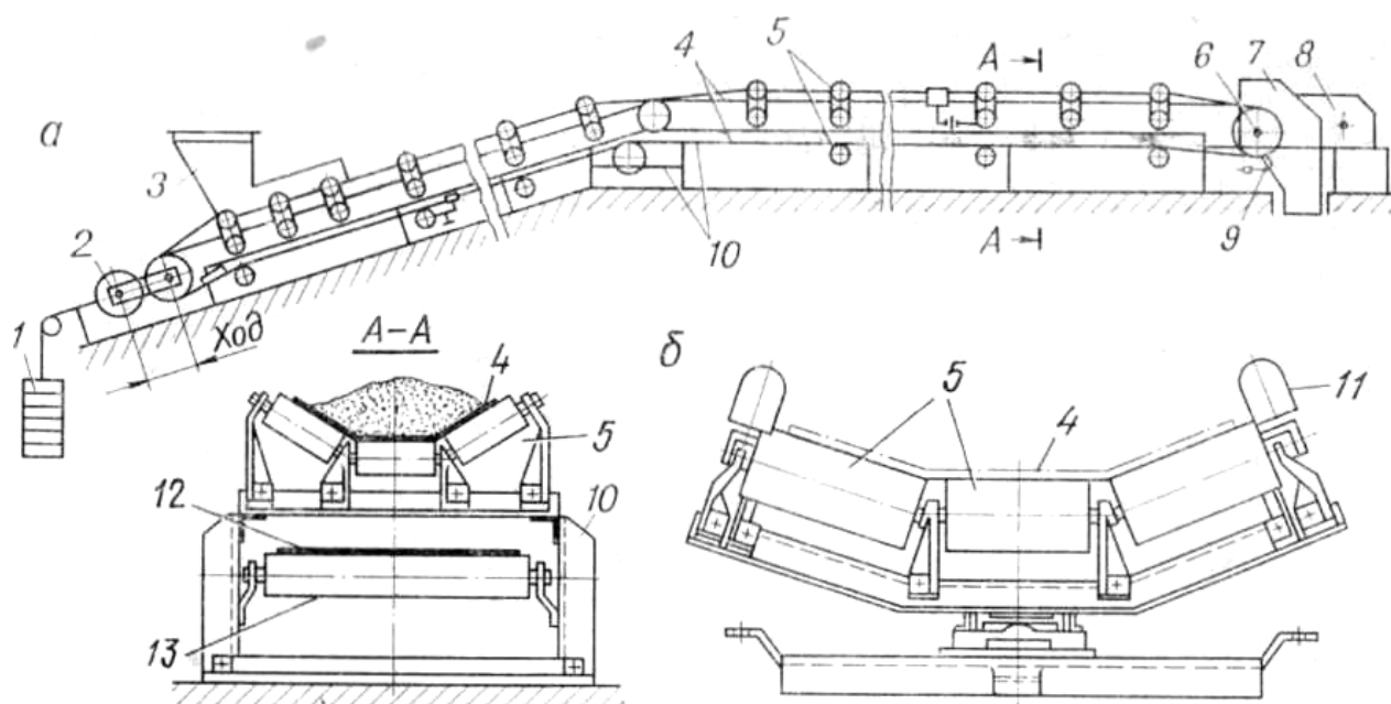
Рис. 11. Стационарный ленточный конвейер:
