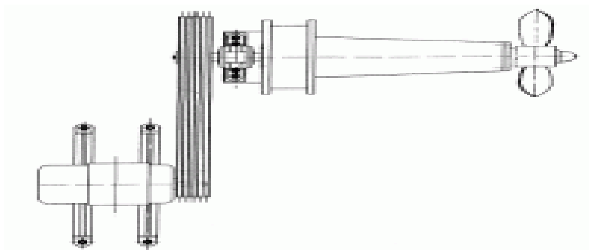
Рис. 6. Чертеж мешалки
