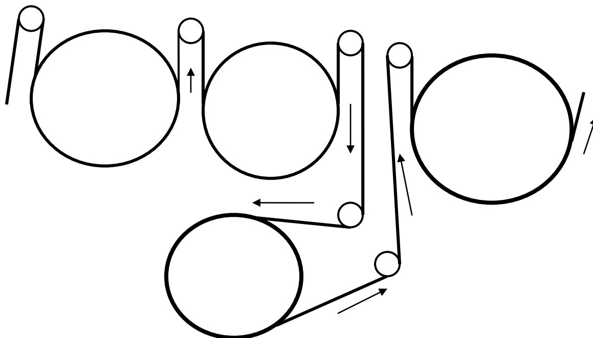
Рис. 7. Схема расположения сукносушителя в прямой ветве сушильной группы
