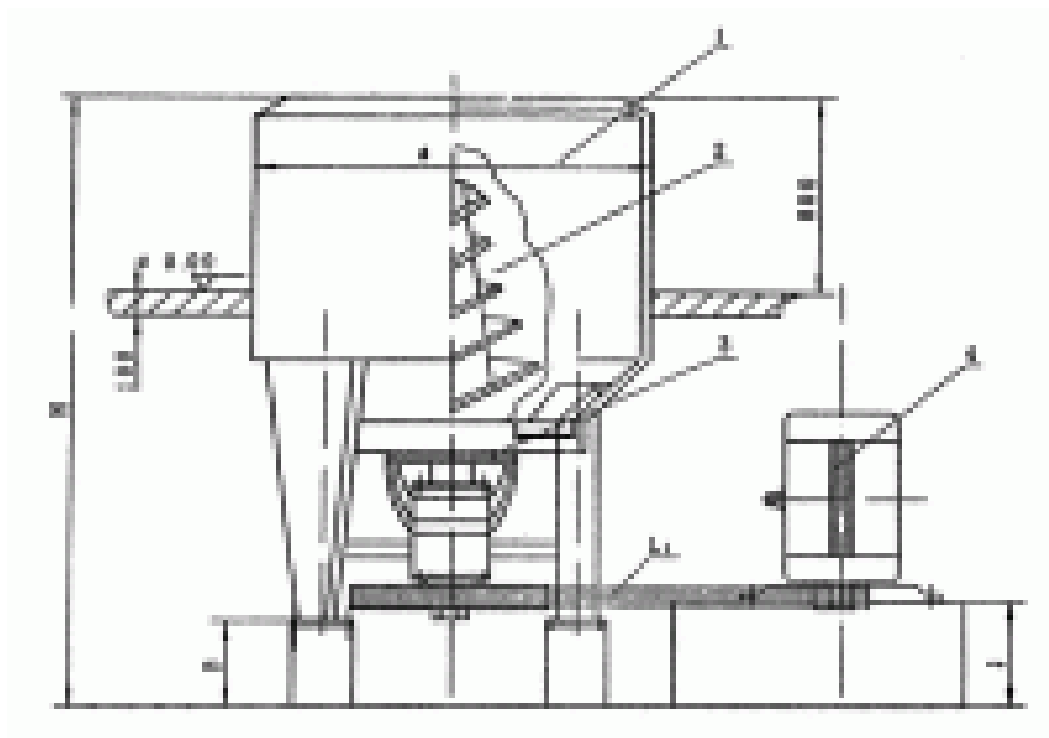
Рис 8. Гидроразбиватель
