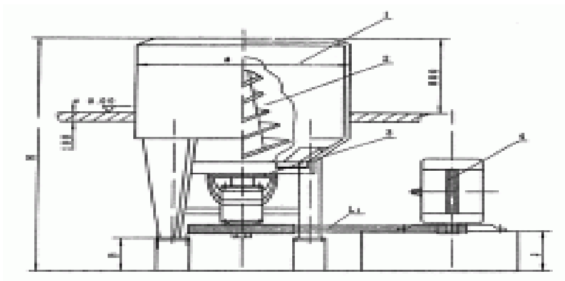
Рис. 2. Чертеж вертикального гидроразбивателя
