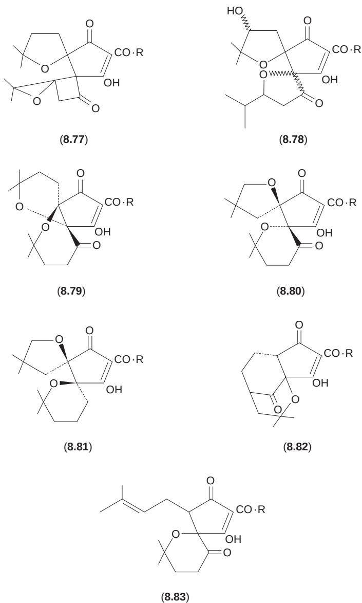
Fig. 8.15 Abeo-iso- \alpha -acids (Verzele and De Keukeleire, 1991).
