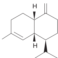
(8.120) γ-Muurelone
