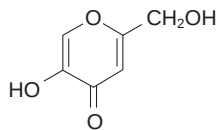
Kojic acid
