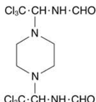
(7.14) Triforine (Saprol)
