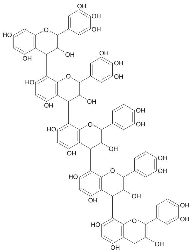
A-prodelphinidin pentamer
