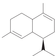
(8.117) α-Muurelone
