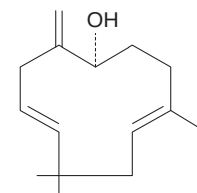
(8.147) humulenol II
