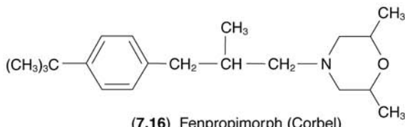
(7.16) Fenpropimorph (Corbel)
