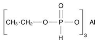
(7.9) Fosetyl Aluminium
