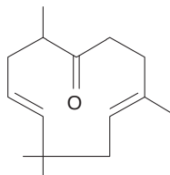
(8.148) humuladienone
