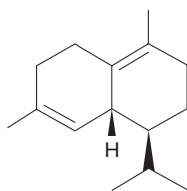
(8.118) δ-Cadinene
