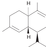
(8.122) α-Cadinene
