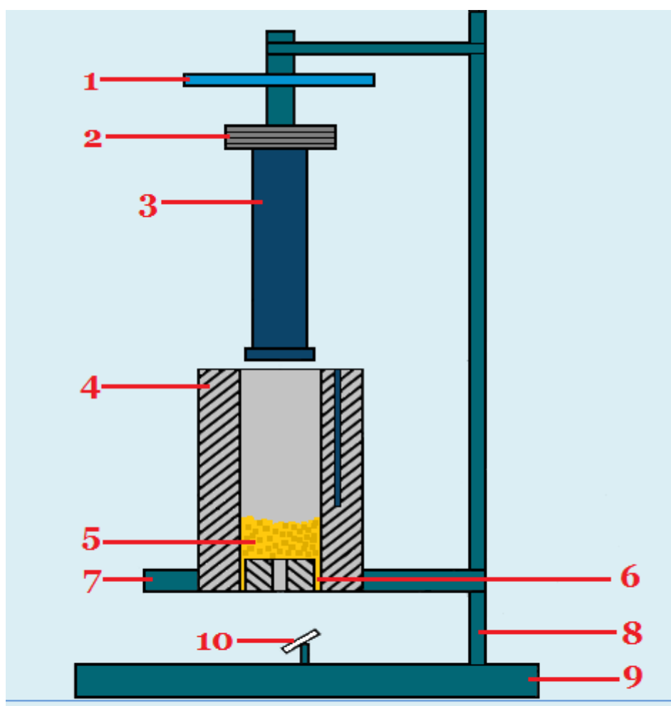
Суёқланма оқувчанлик кўрсаткичини аниқловчи вискозиметрнинг схемаси
