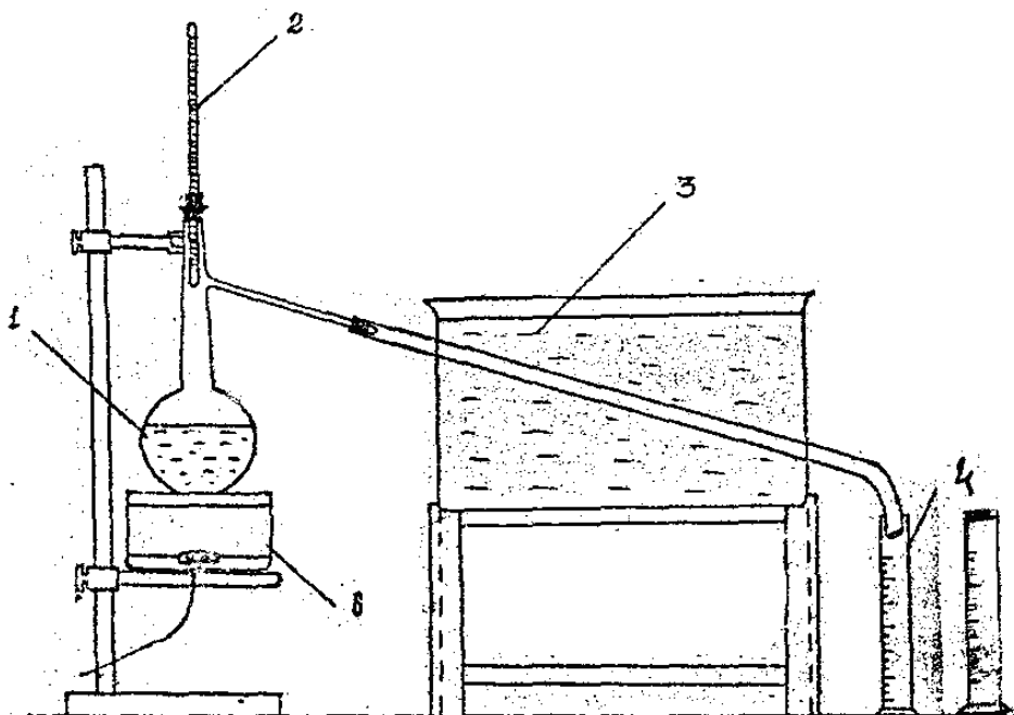
2-расм. Бензиннинг фракцион таркибини аниқлаш асбоби. 1-колба. 2-термометр. 3-совуткич. 4-ўлчамли цилиндр. 5-электроплитка.
