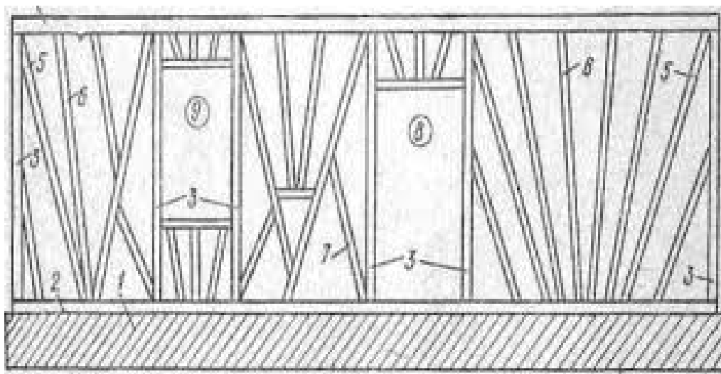
29-расм: Синч девор
