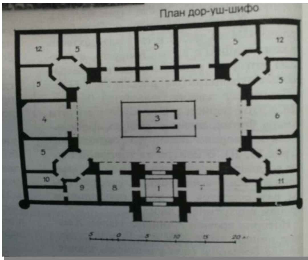
7-расм. Дор-уш-шифо мадрасаси тархи. 17-аср.
