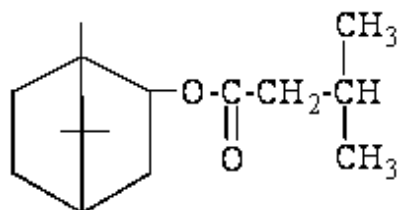
Bornilizovalerianat
