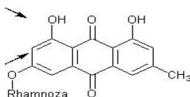
Frangulin A
