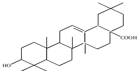
Oleanolol kislota
