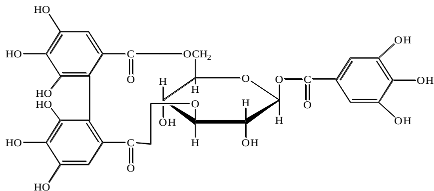
Korilagin
