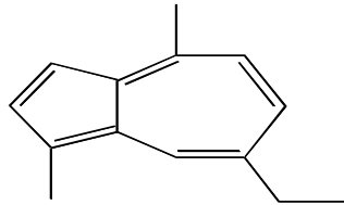
Xamazulen
