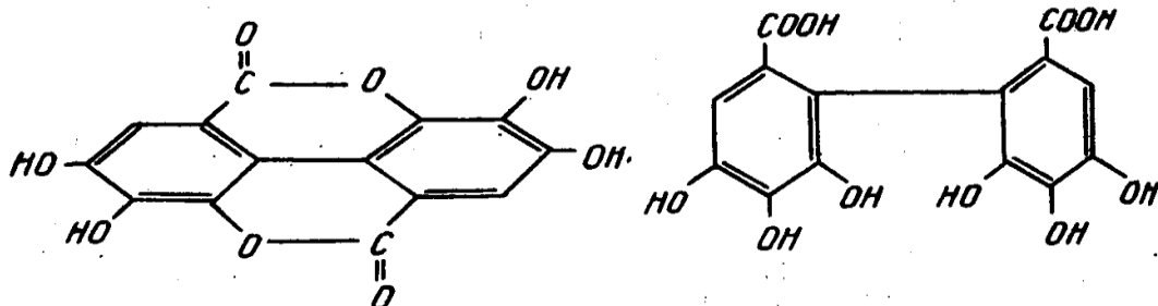
Ellag kislota
