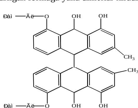
Frangularozid
