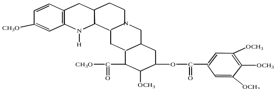
Rezerpin
