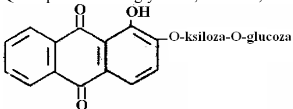
ruberitrin kislotasi
