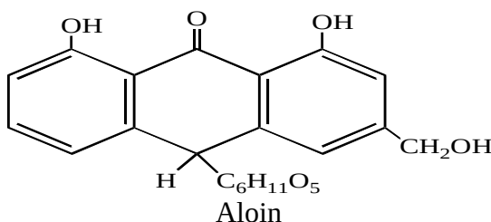
Aloin
