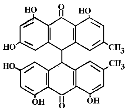
emodindiantron
