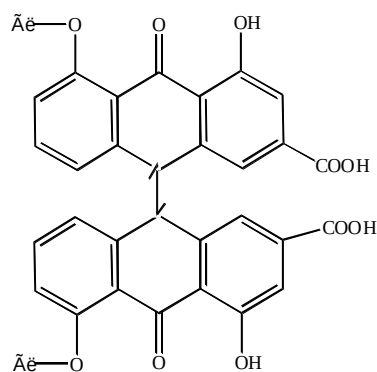
Sennozid A,B
