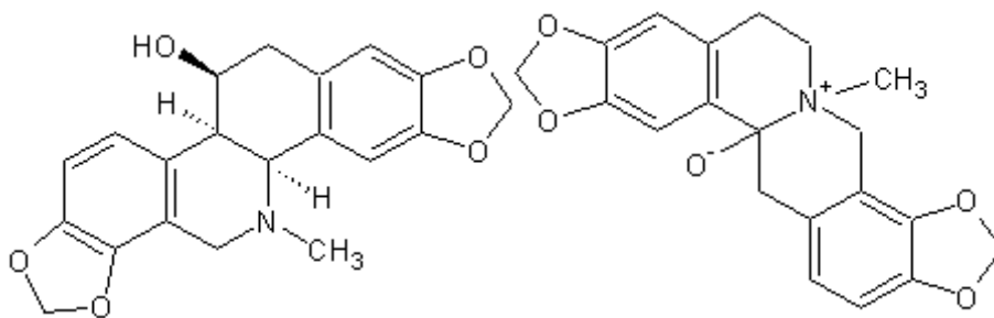
Xelidoiin
