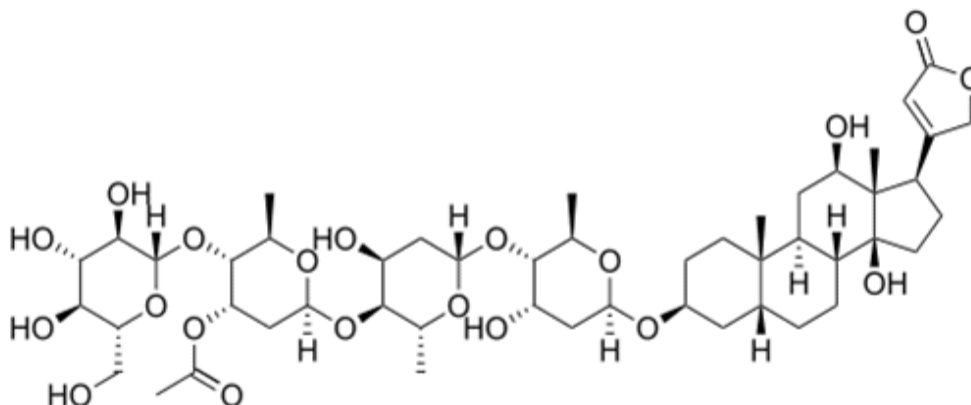
Lantozid C
