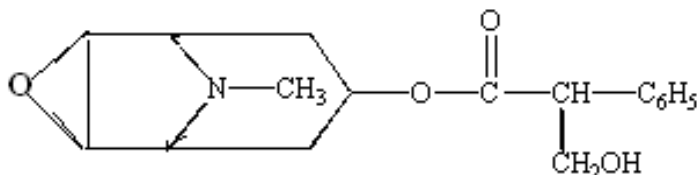
Giostsiamin
