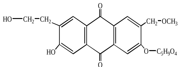
Nataloin
