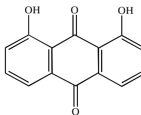
Xriaofanol
