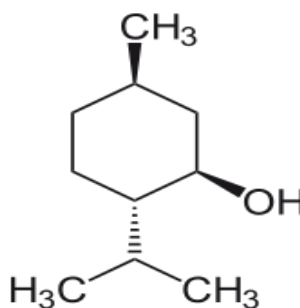
Mentol
