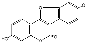
Kumestrol
