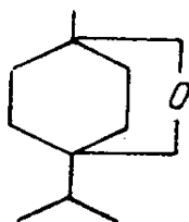
Sineol
