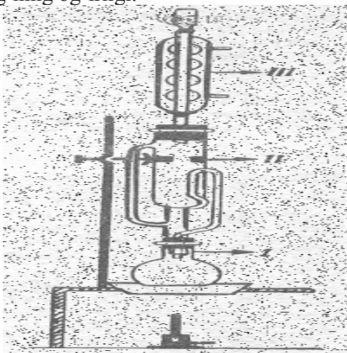
14.1.-rasm. Sokslet apparati.
