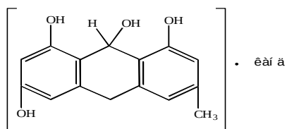
Jesterin
