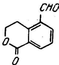
Eritrotsentaurin
