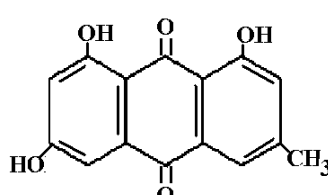
frangula - emodin
