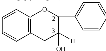
Katexin (3 - flavanol)
