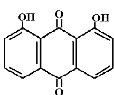
xrizatsin
