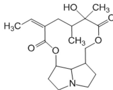
Platifillin
