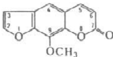
Kantatoksin
