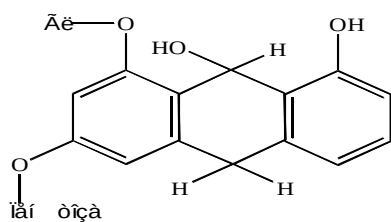
Jesterin
