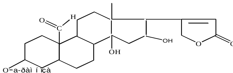
Adonitoksin
