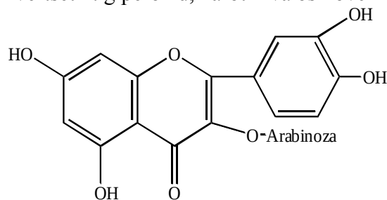
Avikulyarin
