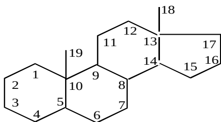
Tsiklopentan pergidrofenantren
