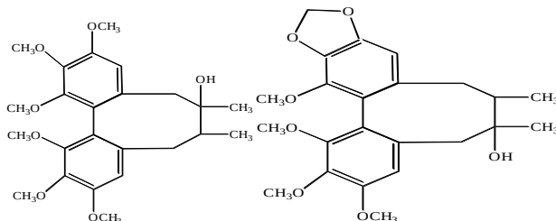
Gomizina
