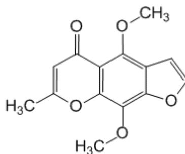
Kellin
