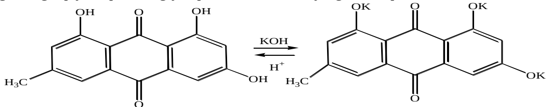
Reum emodin
