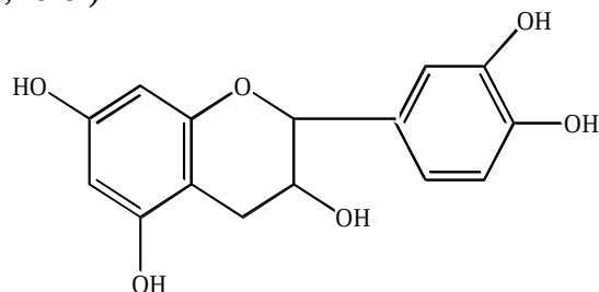
Epikatechin gallat
