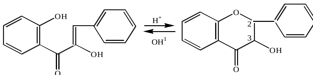
Flavonon
