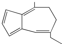
Xamazulen
