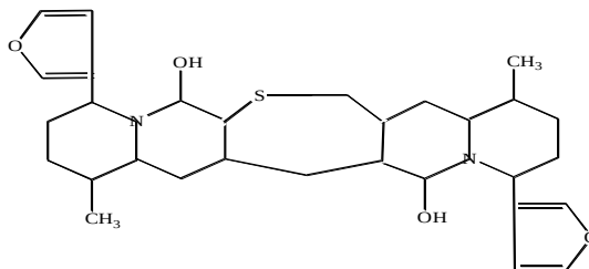
Nuflein
