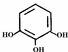
pirogallol
