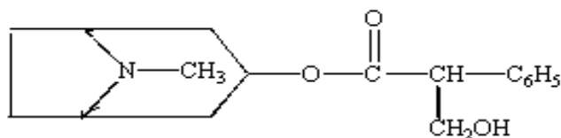
Giostsiamin
