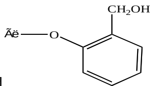
Salitsin
