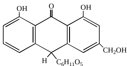
Aloy-emodin-antronni glikozidi
