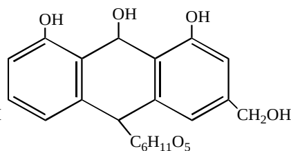
Aloy-emodin-antranolni glikozidi
