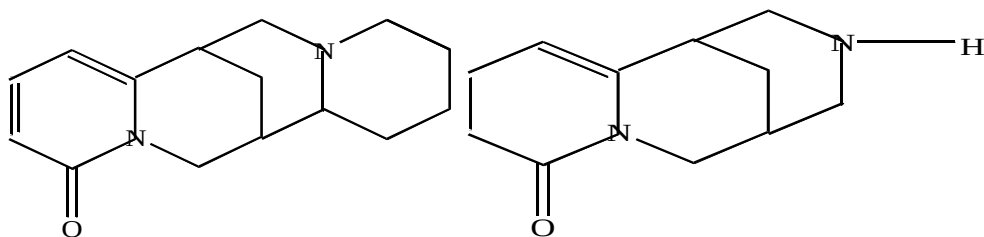
Termopsin
