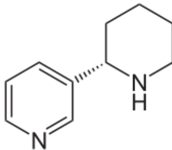
Anabazin
