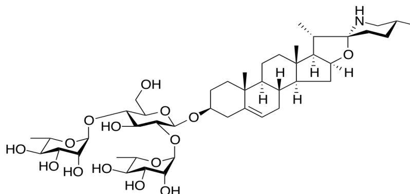
Solamargin
