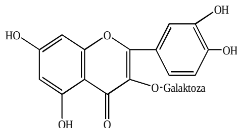
Giperozid
