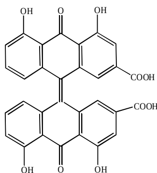
Direin
