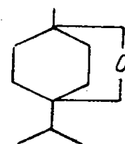
Sineol
