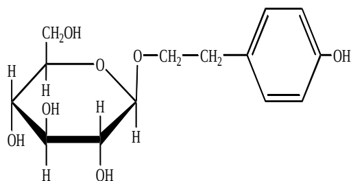
Salidrozd (rodiolozid)
