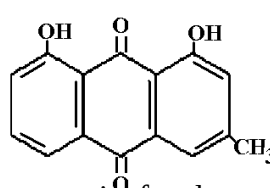
xrizofanol
