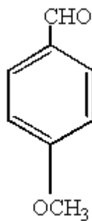
Anis aldegid
