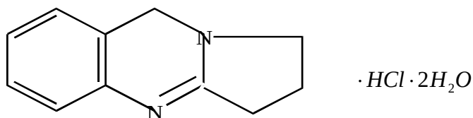
Dezoksipeganin gidrokslorid
