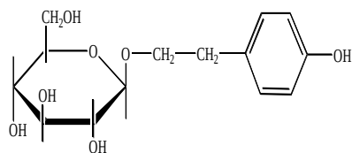
Salidrozyd
