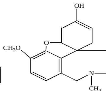
Galantamin
