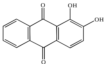
Alizarin
