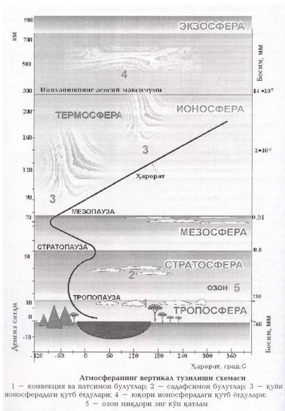
8-расм. Атмосферанинг вертикал тўзилиши ва ҳароратининг юқорига қараб ўзгариб бориш схемаси (Манба. Р.Рамаде, 1998 й.).
