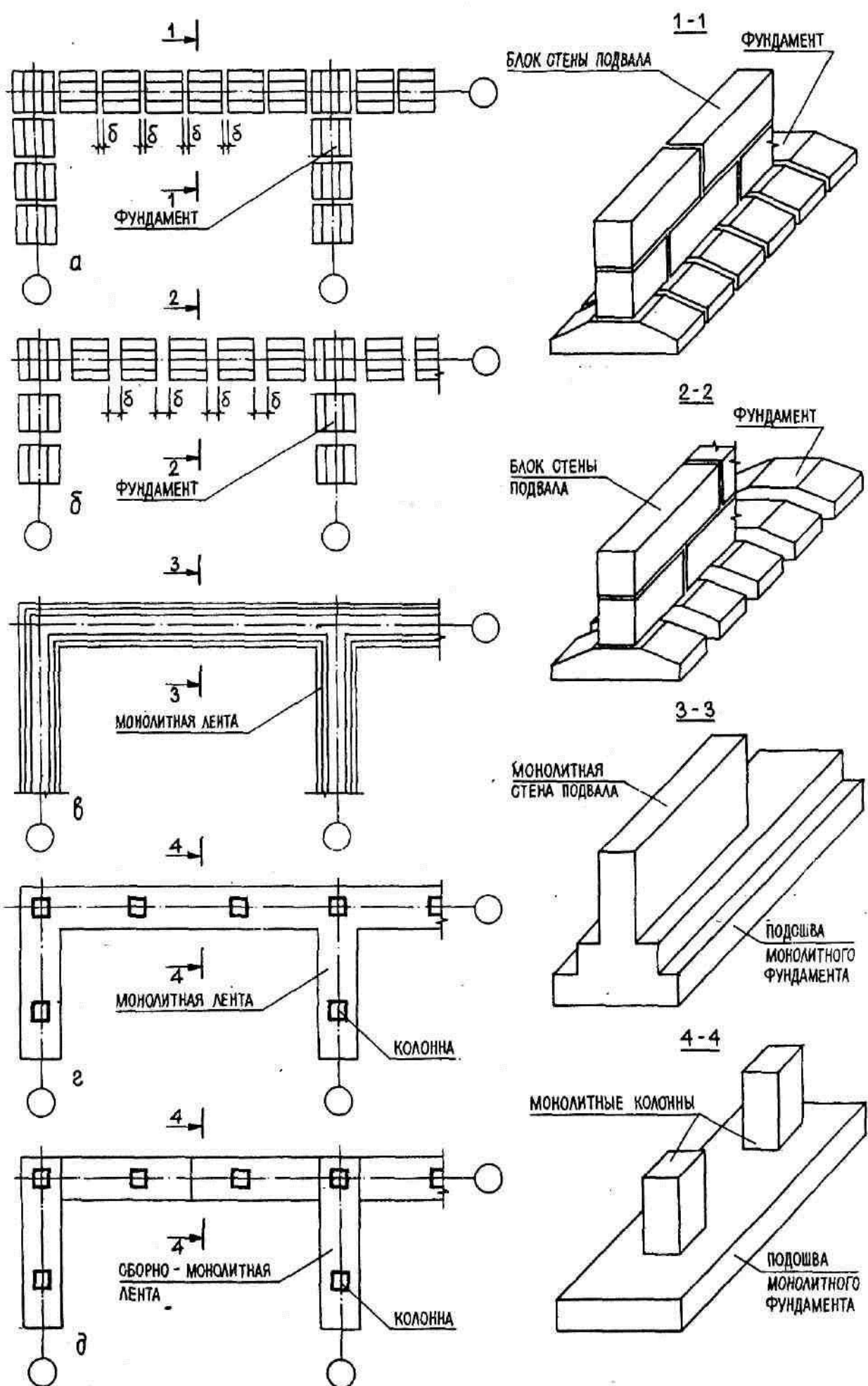
10-рaсм..Лентасимон йиғма-бетон блок ва устунсимон монолит пойдевор.
