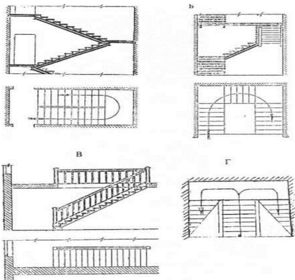
4-расм. А-икки маршли Б-уч маршли В-бир маршли Г-икки маршли (распошная).
