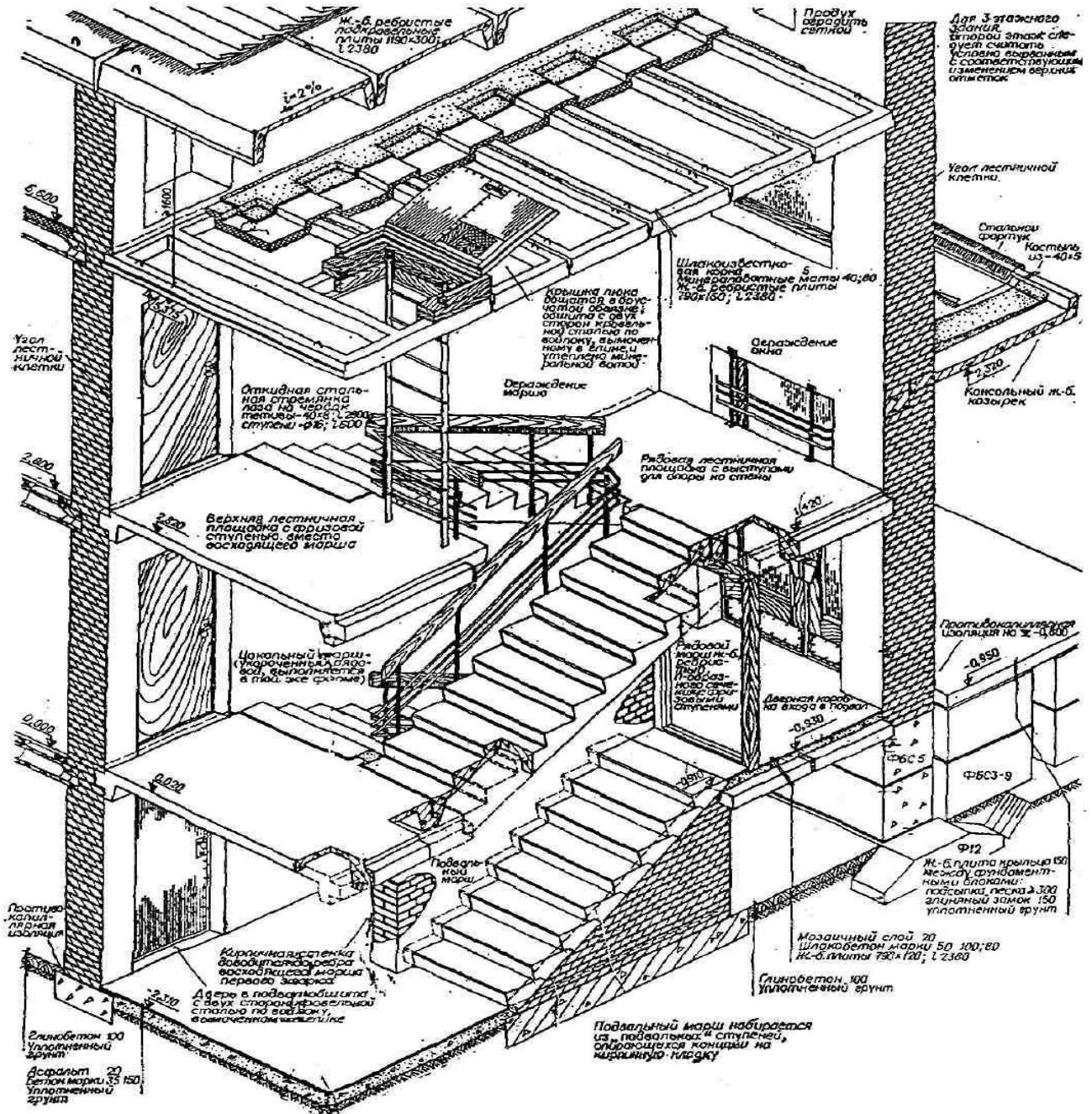
9-расм. Қаватлараро зинапоя майдончаси.
