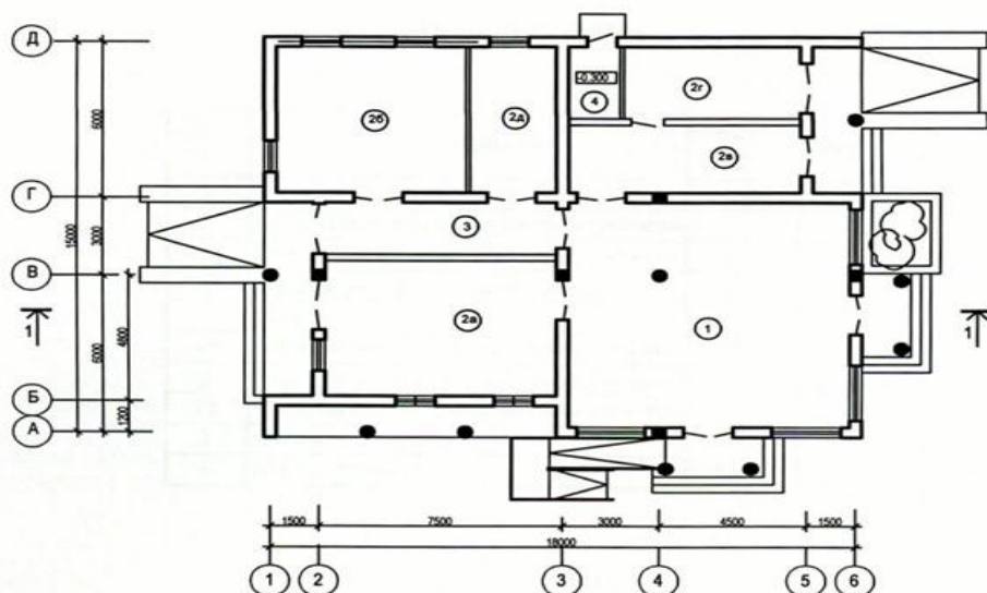
8-расм.ҚУРИЛИШ ҚУРИЛИШ МАТЕРИАЛЛАРИ ДЎКОНИ БИНОСИ.
