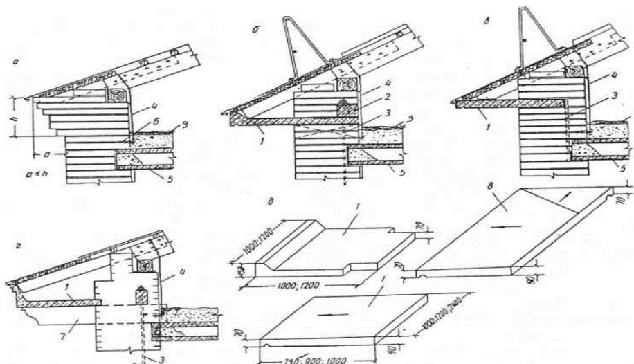
12-расм. Том ёпма конструктив элеменларнинг тугунлари.
