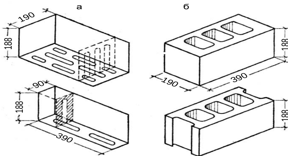
7-расм. Енгил бетон майда блоklar:
