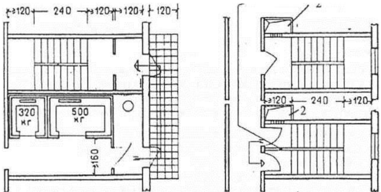
5-расм. Тутун кирмайдиган зинахоналарнинг типлари:
