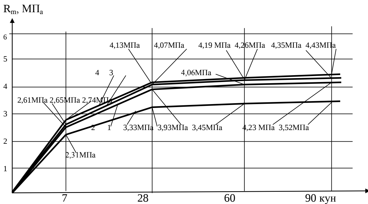
3.6-расм. Вермикулитбетоннинг вақт бўйича призмавий мустаҳкамлигининг орттиш графиклари. 1-бетон призма; 2-3-4-волластонит қўшилмали призма.
