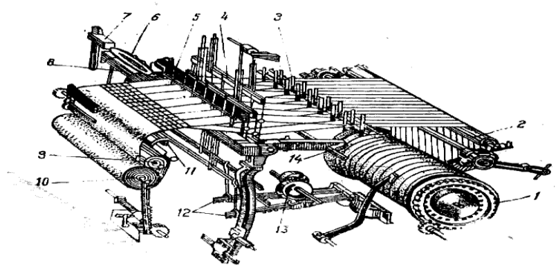
9-rasm. To'quv dastgohining umumiy ko'rinishi.
