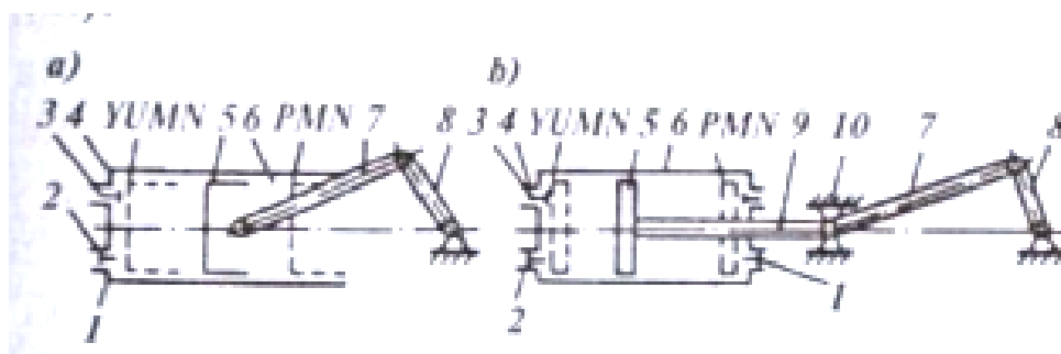
1- расм. Поршенли компрессор схемиси: а) крейскопфсиз оддий ҳаракатли; б) - крейскопфли иккиламчи ҳаракатли. 1 - кўтариш клапани; 2, 4 - кўтариш ва сўриш патрубкasi; 3 - сўриш клапани; 5 - поршен; 6 - цилиндр; 7 - шатун; 8 — коленчат вал кривошипи; 9 - шток; 10 - крейскопф; YUMN - юқориги «мавхум» нуқта; PMN - патски «мавхум» нуқта.
