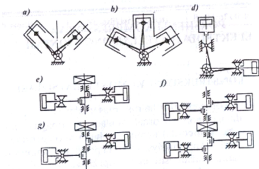
2- расм. Кўр поғонали компрессорлар цилиндрларининг жойлашуви бўйича принципиал схемалари: a - V -- ҳолатдаги; b - W- ҳолатдаги; d - вертикал ҳолатдаги; e, f, g - горизонтал оппозит ҳолатдаги.
