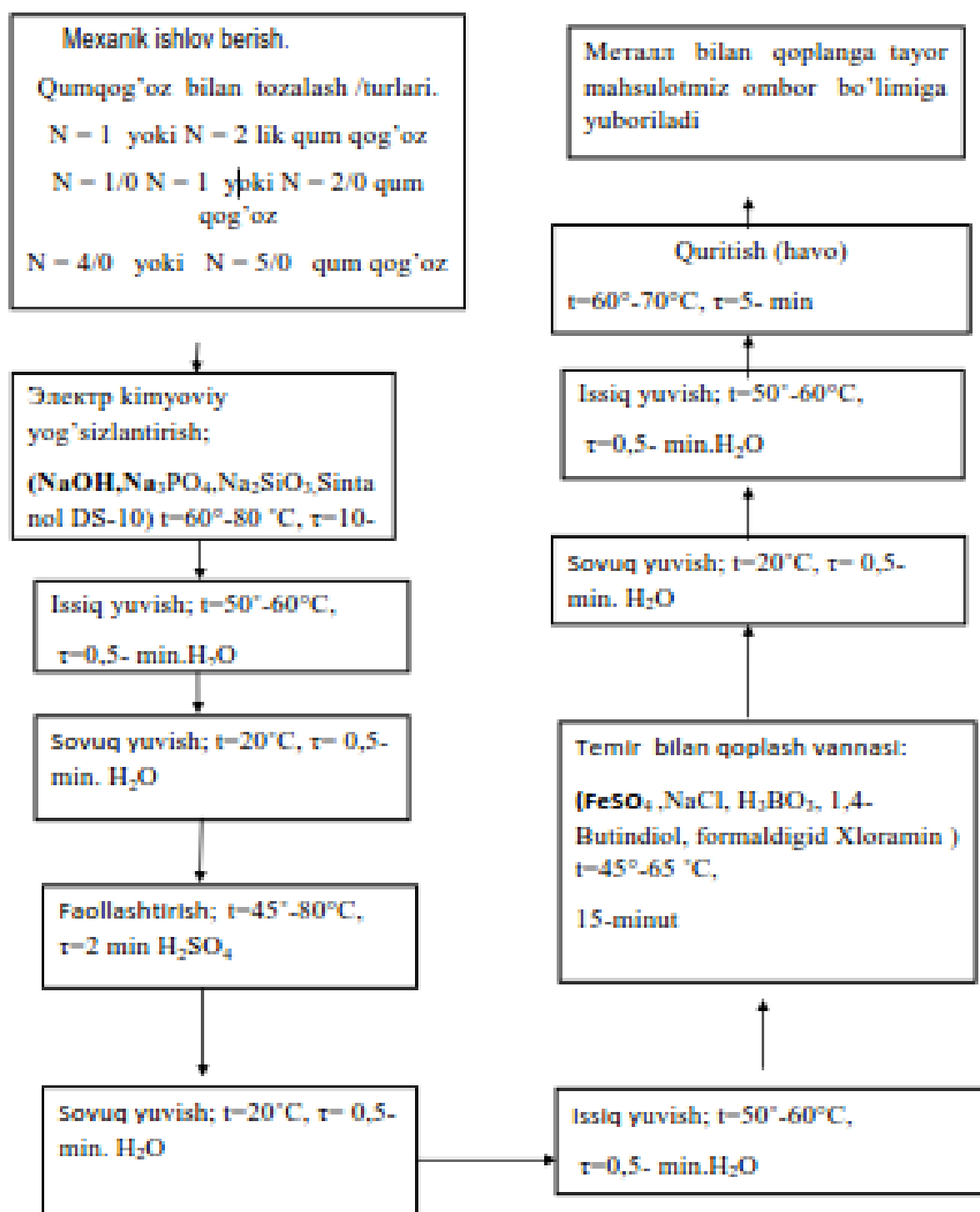
Galvanik qoplash texnologik sxemasi. 2-jadval.
