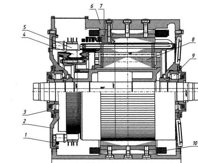
Рисунок 2 – Тяговый электродвигатель электровоза «Синара»
