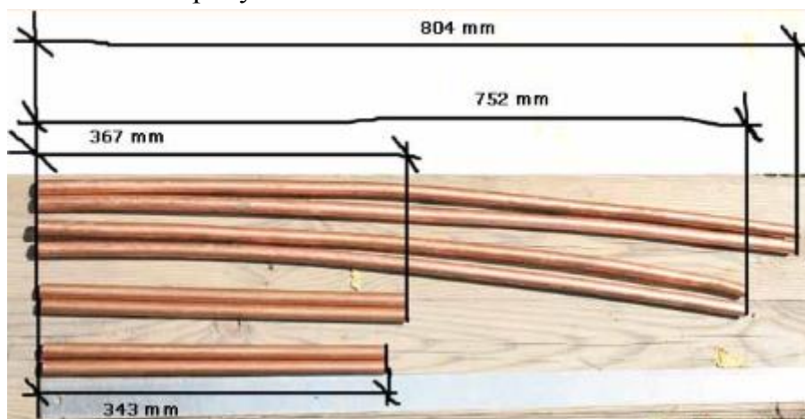
Рисунок 1 – Размеры медных труб
