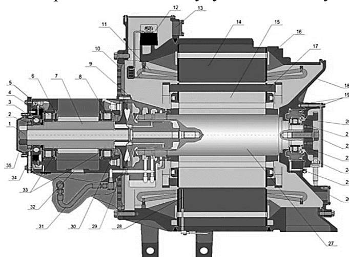
Рисунок 1 – Тяговый электродвигатель электровоза «Гранит»
