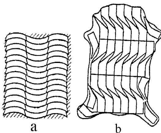
Rasm 2.3. Andozalararo chiqindilar chiqmaydigan qiyshiq chiziqli qism andozalarining shakli
