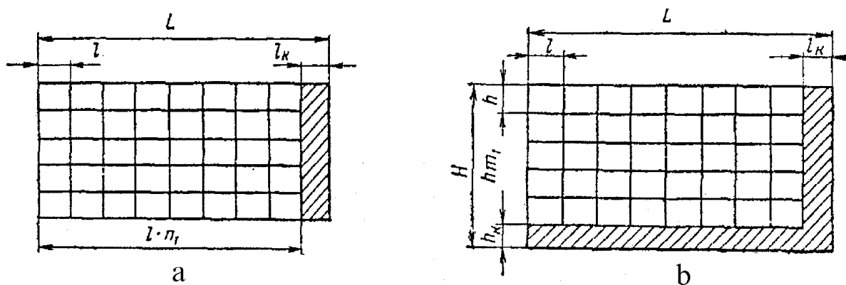
Rasm 2.7. To'g'riuchakli andozalar va bichiladigan materiallarni qaytarilmaydigan razmerlari
