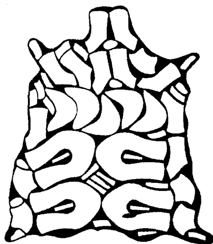
Rasm 5.12. Ayllarning poshnasi qoplangan yaxlit qisimli «lodochka» tuflisini, maktab qizlarining tuflisini qismlari bilan birgalikda, II nav shevrodan bichilgan tasviri
