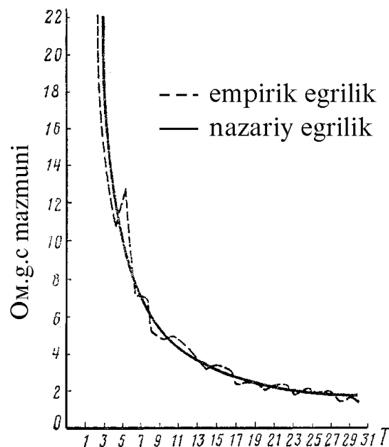
Rasm 2.12. Nuqsonlarni tarqalishi T=W/\Sigma g\sqrt{n} va O_{gc} chiqindilar orasidagi bo'g'liqliq egri chizig'i
