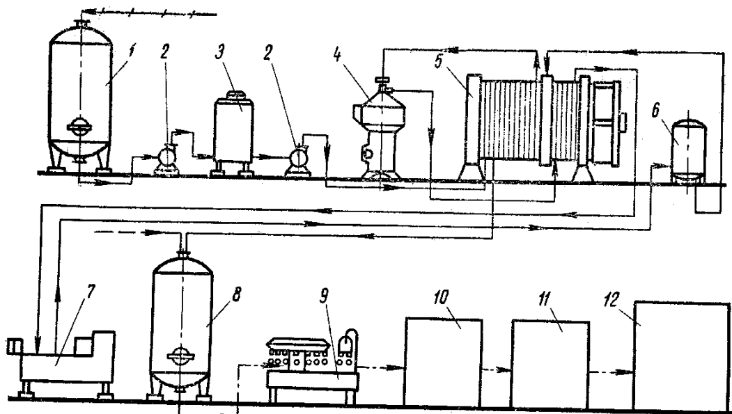
1-rasm. Termostat usulida sut-achitqi mahsulotlarini ishlab chiqarish texnologik sxemasi.
