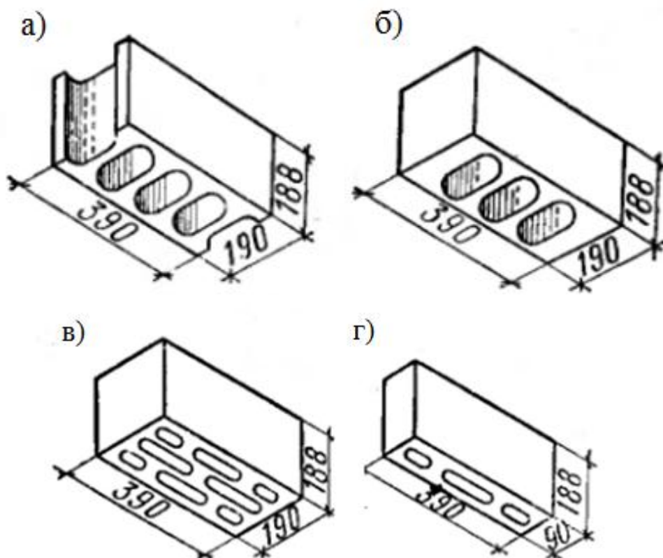
Рис.5. Мелкие легковесные стеновые блоки: а – трехпустотный ложковый ; б – то же, тычковый; в – щелевидный; г – доборная половинка [2].
