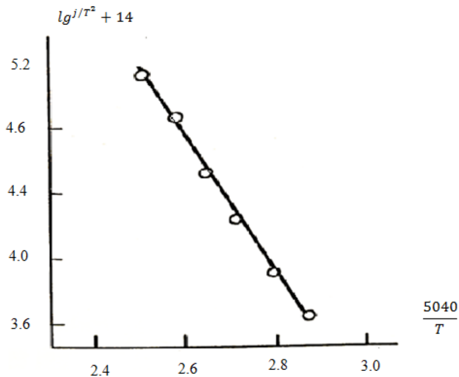
3.1.5-расм. Молибденнинг (111) қиррасининг \lg J/T^2 = f(5040/T) боғлиқлиги Ричардсон тўғри чизиғи ( e\varphi_R = 4,18\pm 0,05 эВ)
