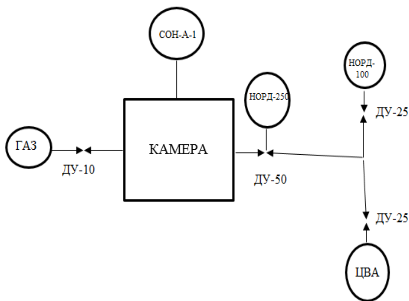
2.4.1-расм.Вакум тизимининг блок схемаси
