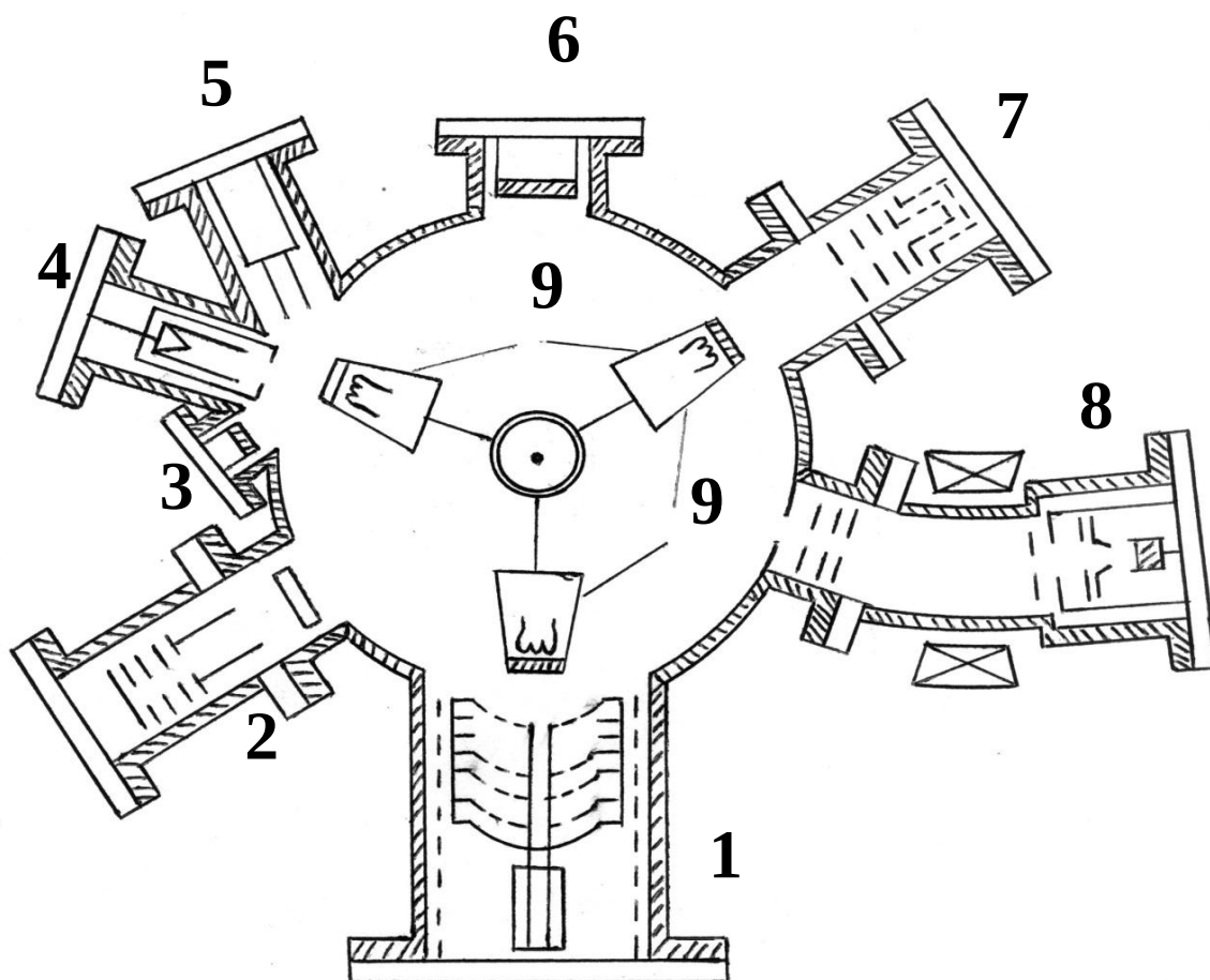
2.2.2-расм. Экспериментал қурилма ишчи камерасининг схематик кесим кўриниши.
