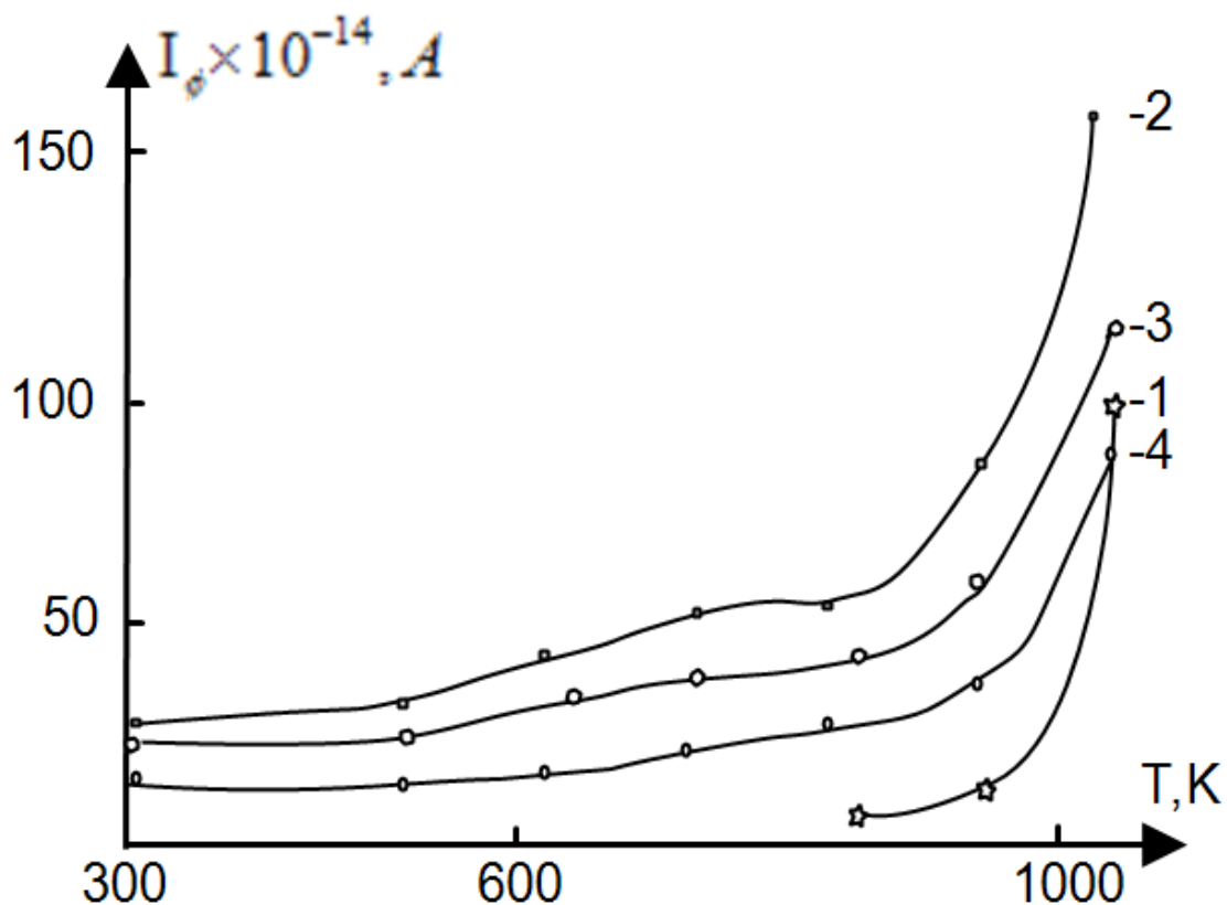
3.2.1-Расм Фотоэмиссион токнинг температурвий боғлиқлиги эгри чизиқларинг берилиши 4,66эВ (1) , 4,87эВ (2) ва 5,15эВ (3) 4-термоток
