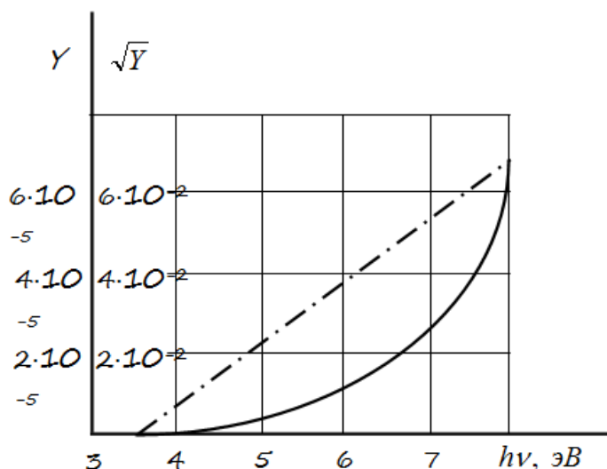
1.2.1–расм. Металлнинг квант чиқиши Y(h\nu) нинг спектрга боғлиқлиги ва фотозффе́кт бўсағасини (чиқиш ишини) график аниқлаш
