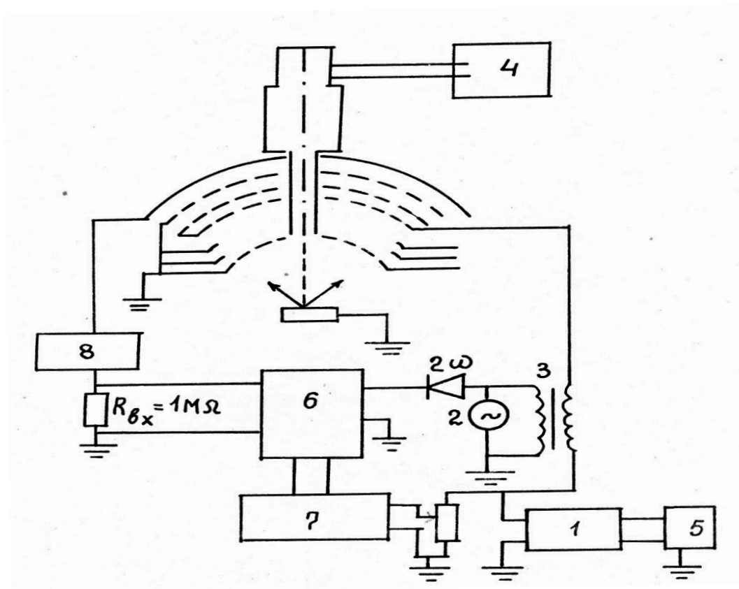
4-расм. Оже- сигналларни қайд этиш блок схемаси.
