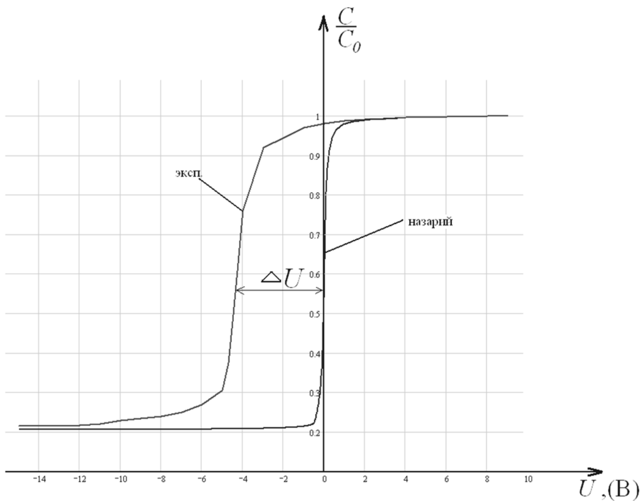
3.3-рasm: МДЯ – структуранинг диэлектрик қатлам сифими катталигига нормаллаштирилган экспериментал ва назарий вольт–фарада характеристикаларини солиштириш
