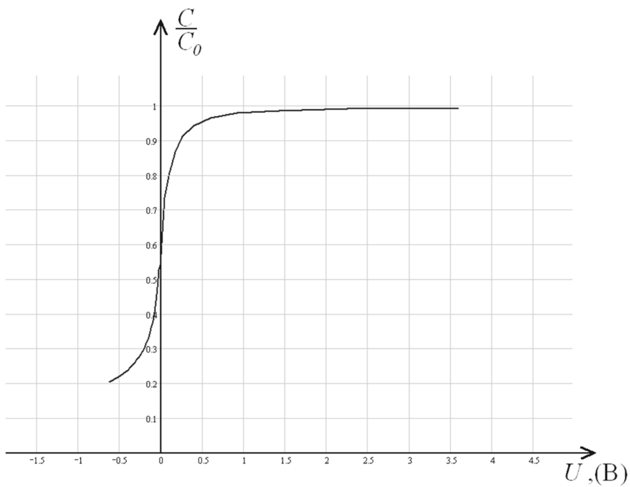
3.2-расм: МДЯ – структуранинг назарий вольт–фарада характеристикаси
