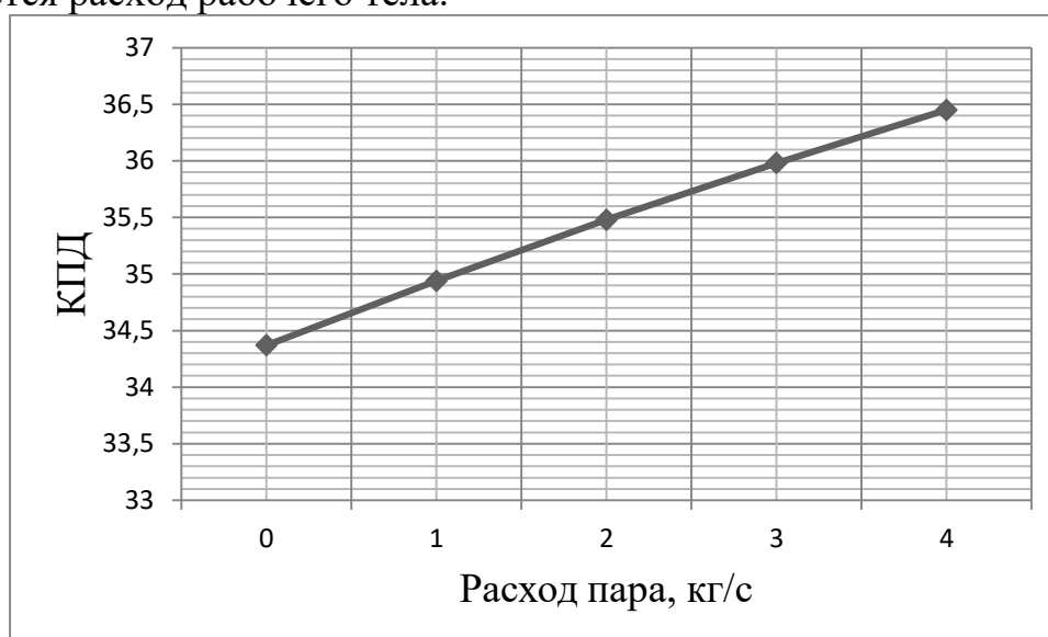
Рисунок 5.3 – Зависимость КПД ГТУ от расхода пара
