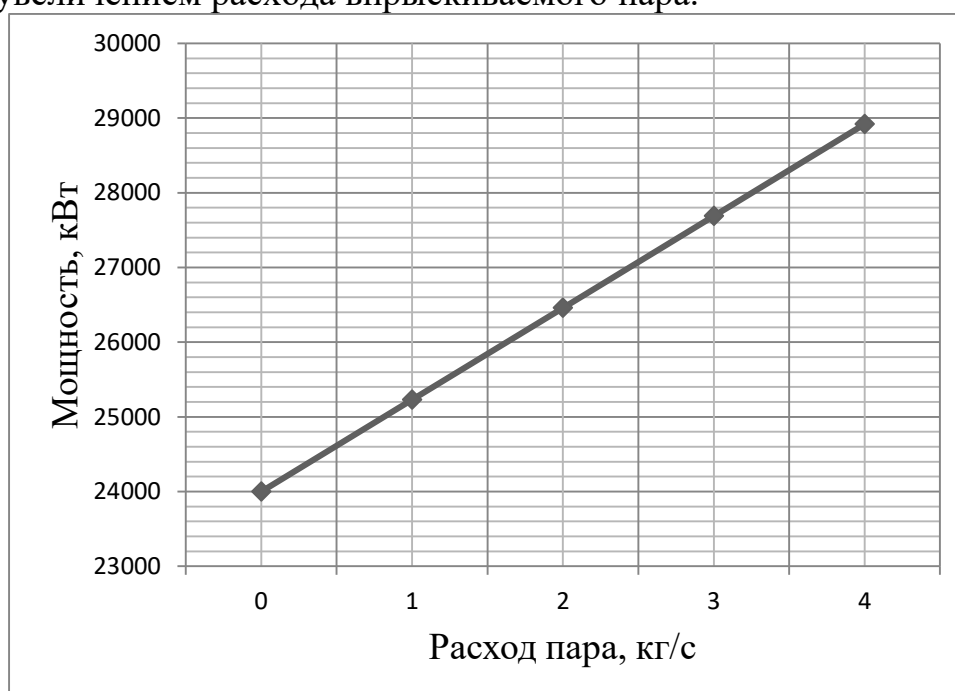
Рисунок 5.2 – Зависимость мощности ГТУ от расхода пара
