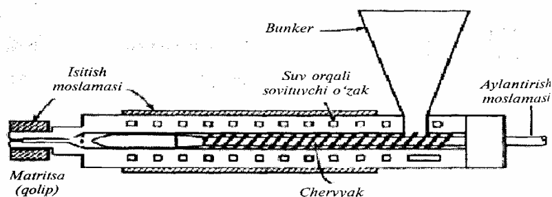
2-rasm. Ekstruder sxemasi
