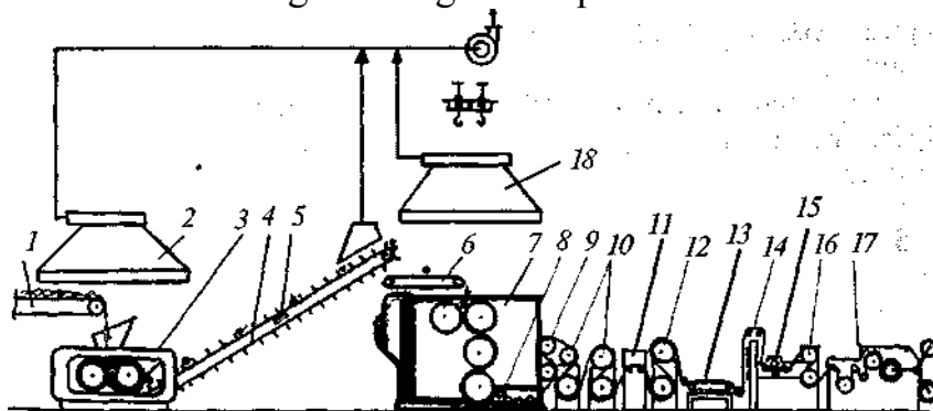
1-rasm. Kalandrlash usulida PVX plyonkasini ishlab chiqarish texnologik sxemasi
