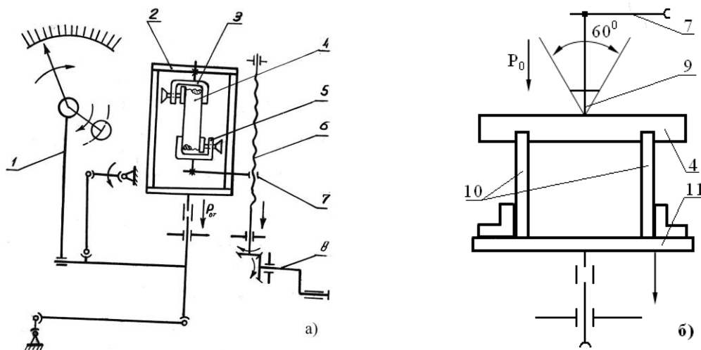
1-расм. Пояларни узиш (а) ва эгиб-синиш (б) кучларини ўлчов асбоби тасвири
