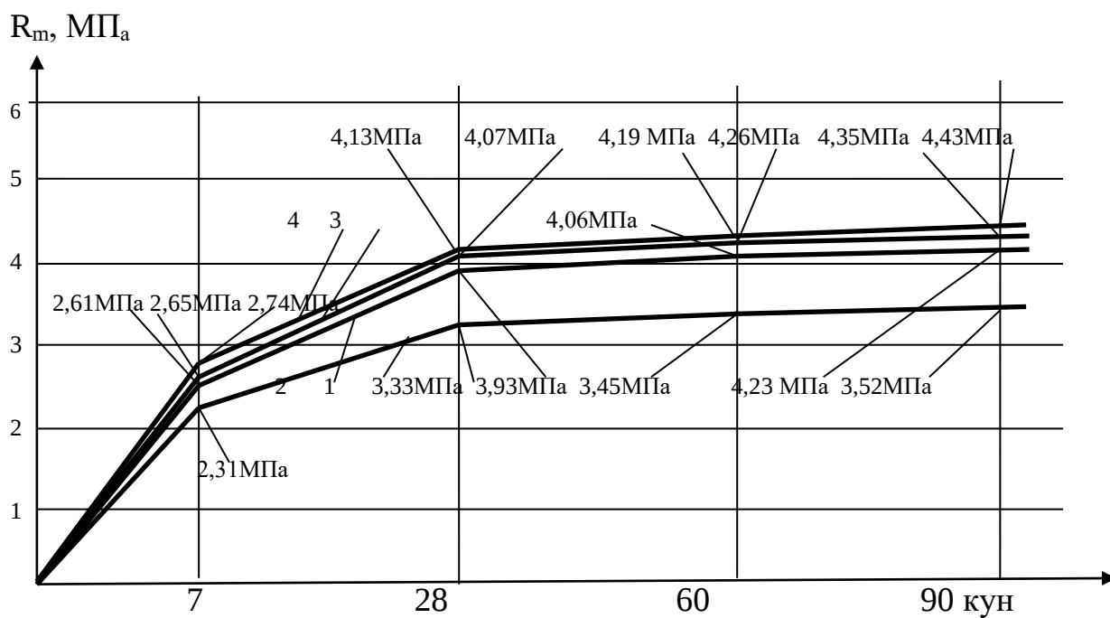
3.6-расм. Вермикулитбетоннинг вақт бўйича призмавий мустаҳкамлигининг ортиш графиклари. 1-бетон призма; 2-3-4-волластонит қўшилмали призма.
