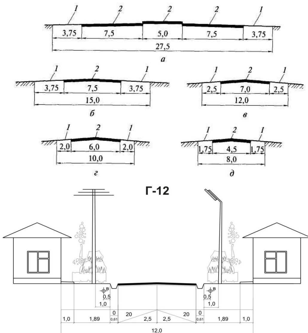
Qishloq tezkor yo'llarining ko'ndalang kesimi (yo'lining yarmi ko'rsatilgan).
