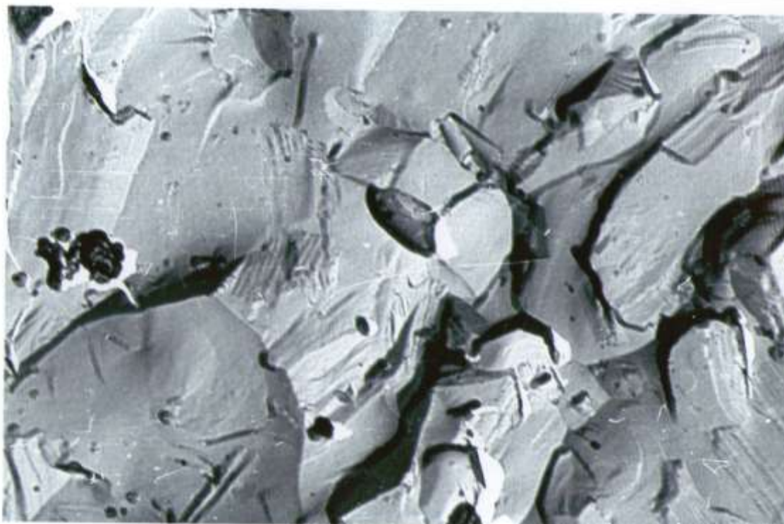
Расм 3.2. “Цемент+сув” таркибли портландцемент тошининг электрон-микраскоп ёрдамида 5600 марта катталаштирилган ҳолати
