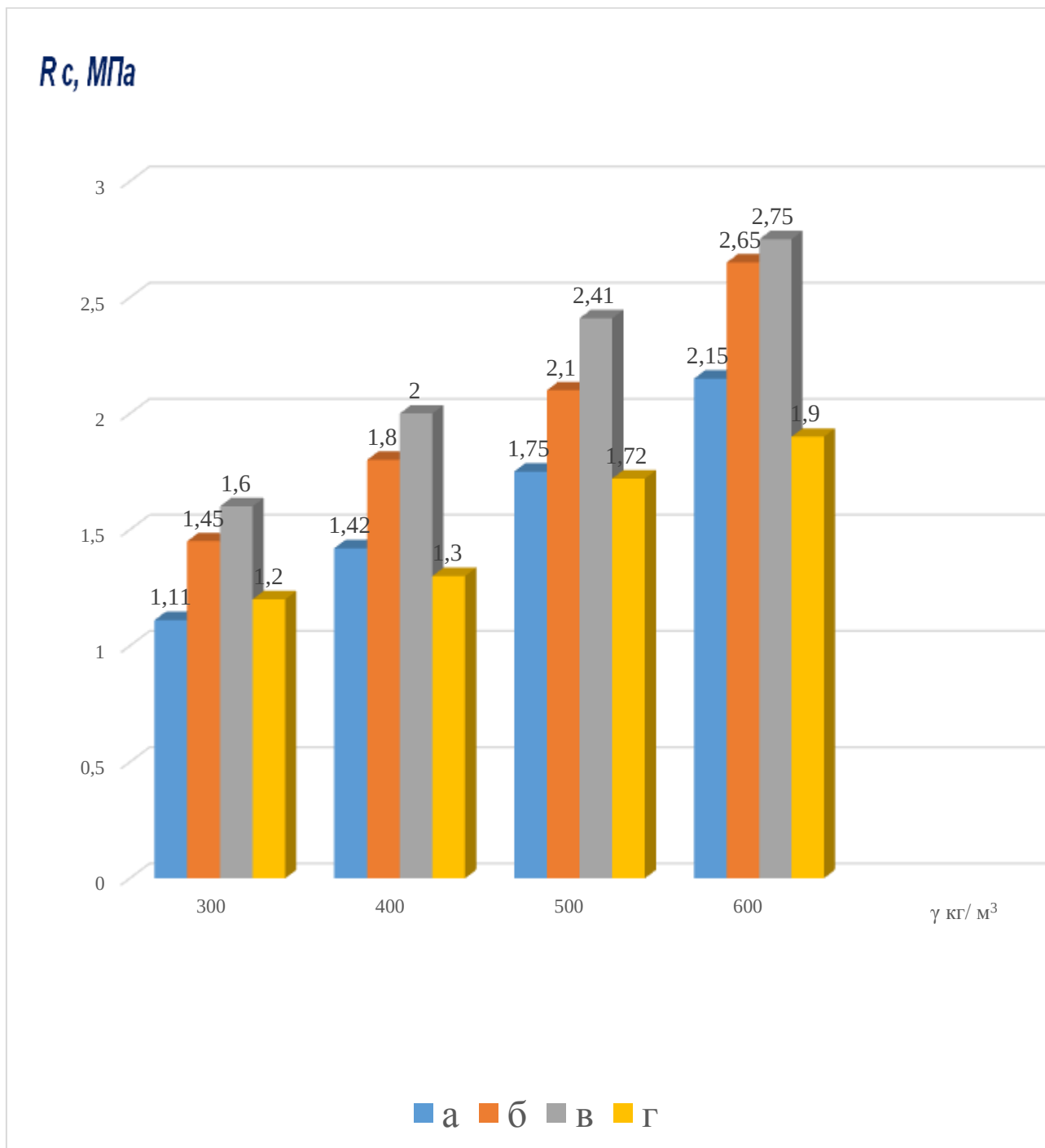
График 3.3. Ишқорли кўпикбетон муштаҳкамлигининг ўртача зичликга боғлиқлиги.
