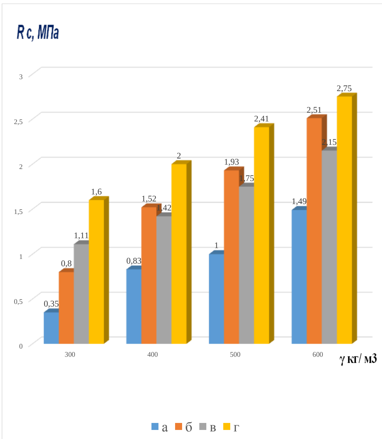
График 3.4. Кўпик бетонларнинг мустахкамлигининг боғловчи моддалар турига боғлиқлиги.
