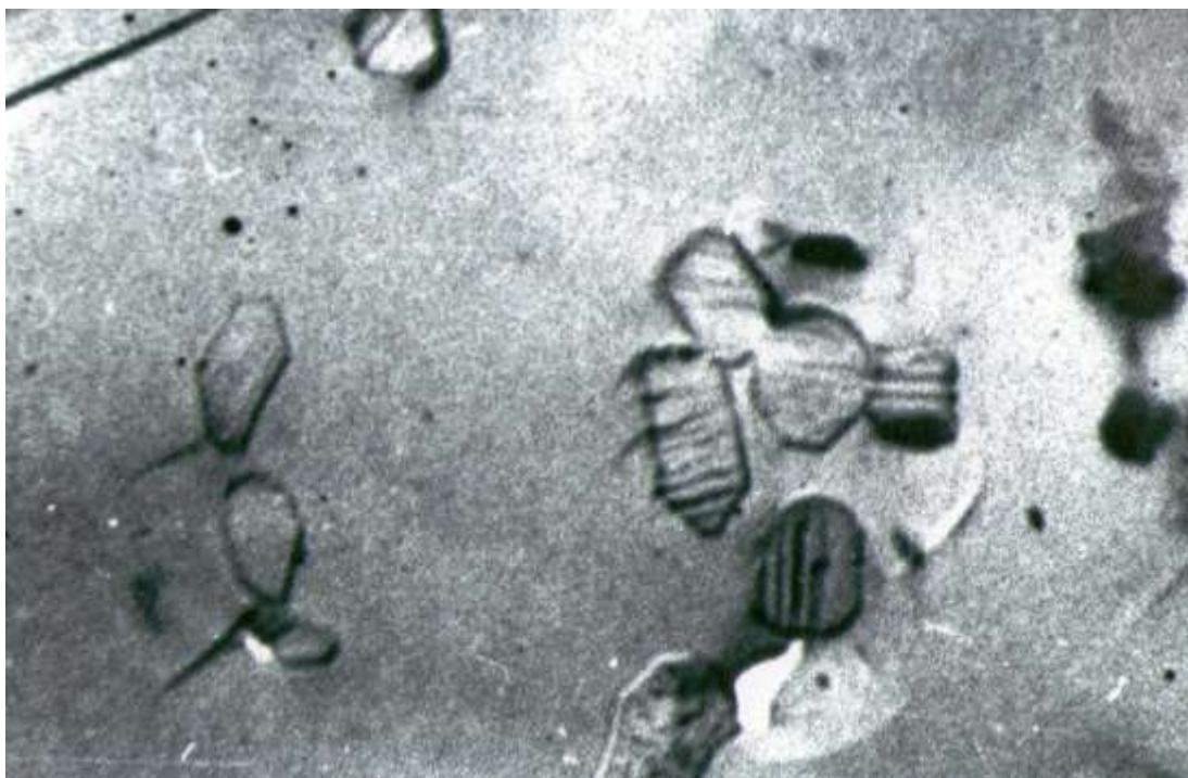
Расм 3.1. “ЭТФ шлаги+Суюқ шиша” таркибли ишқорли цемент тошининг электрон-микраскоп ёрдамида 5000 марта катталаштирилган ҳолати.
