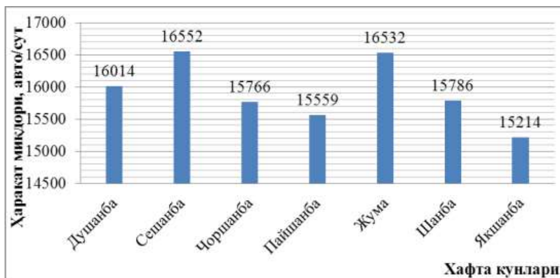
14-rasm Harakat miqdorining hafta kunlari bo'yicha o'zgarish gistogrammasi.
